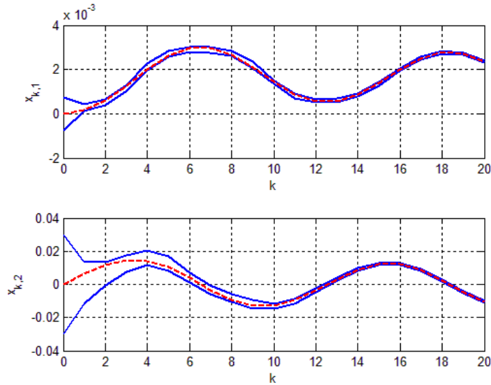
Рис. 4. Результаты гарантированного оценивания в случае, когда известен вид разложения возмущений w_k (пунктир – истинное значение вектора состояния, сплошная линия – граница множественных оценок) Fig. 4. Set-valued estimates when the disturbance w_k decomposition model is known (dashed line denotes the real value of state vector, solid line shows the borders of set-valued estimates)
