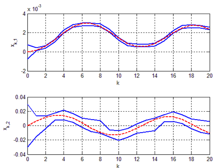
Рис. 3. Результаты гарантированного оценивания в случае, когда известно только множество возможных возмущений W (пунктир – истинное значение вектора состояния, сплошная линия – граница множественных оценок) Fig. 3. Set-valued estimates when only the set of disturbance possible values W is available (dashed line denotes the real value of state vector, solid line shows the borders of set-valued estimates)
