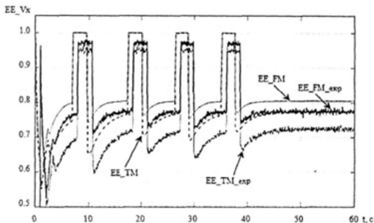
Рис. 6. Расчетные ( EE_{FM} , EE_{TM} ) и экспериментальные ( EE_{FM_{exp}} , EE_{TM_{exp}} ) значения энергоэффективности автомобиля УРАЛ-43203 при определении времени разгона до 60 км/ч на типовых ( TM ) и форсажных ( FM ) режимах работы МТУ
