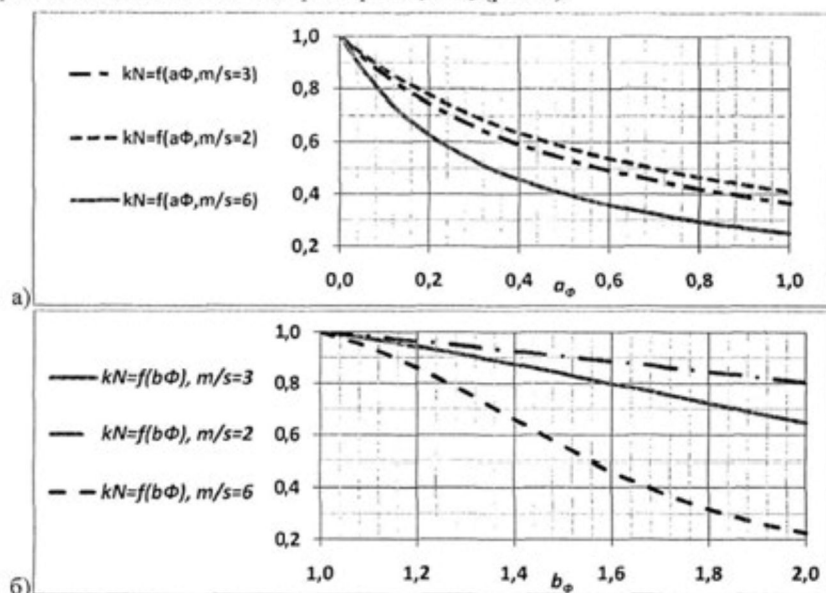
Рис. 4. Влияние факторов a_\Phi и b_\Phi на коэффициент k_N :
