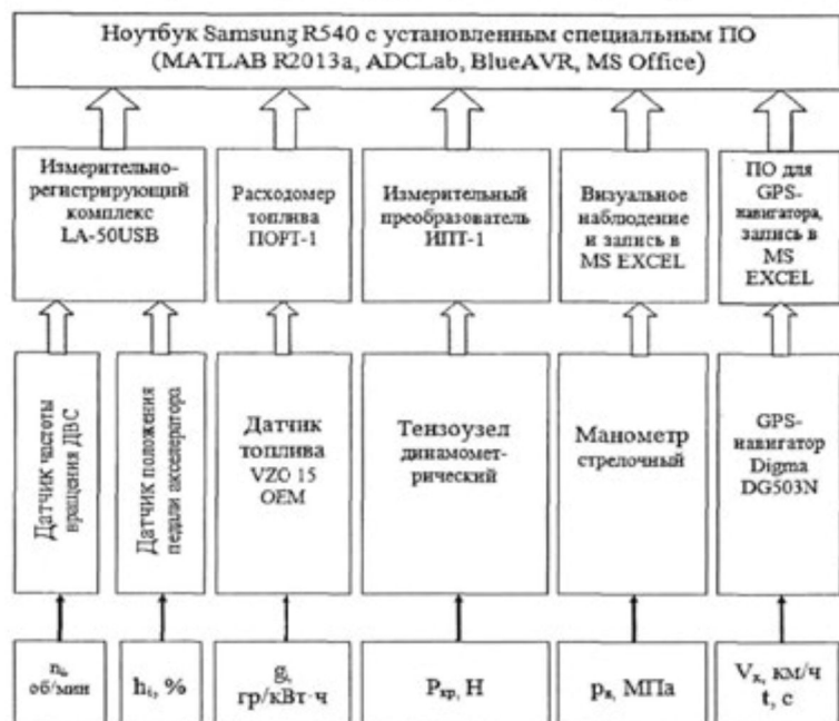
Рис. 5. Структурная схема измерительно-регистрирующей системы
