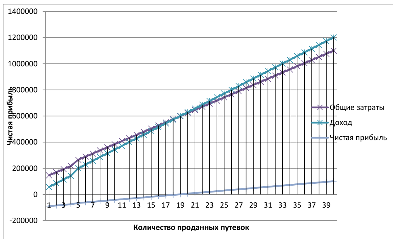
Рисунок 2 – Точка безубыточности
