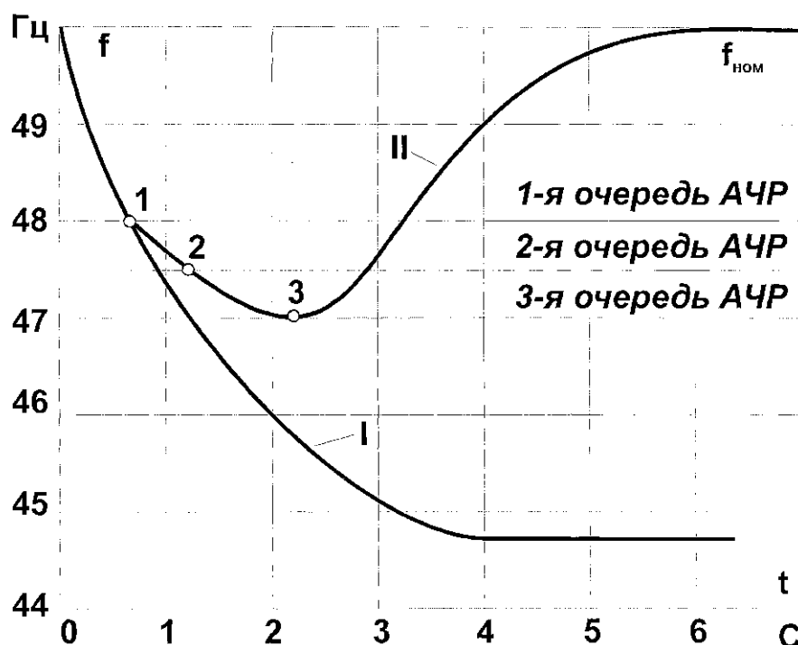
Рис. 1. Процесс изменения частоты в энергосистеме, при дефиците мощности
