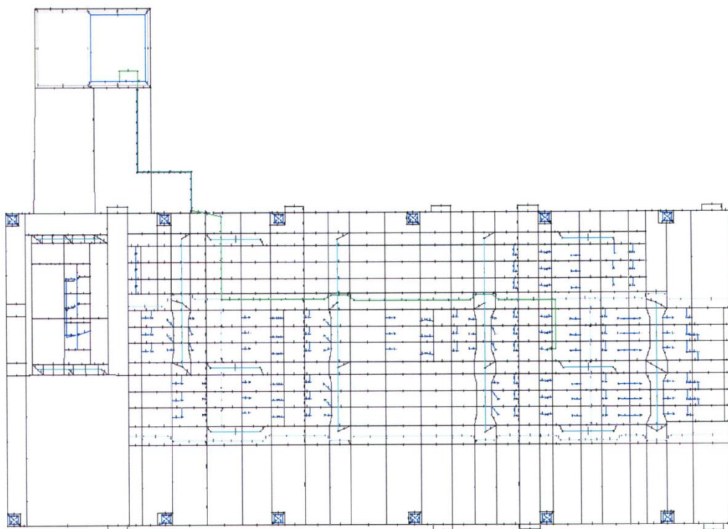
Рисунок 3- Расчетная схема ЗУ ОРУ 220 кВ в программе ОРУ-Проект
