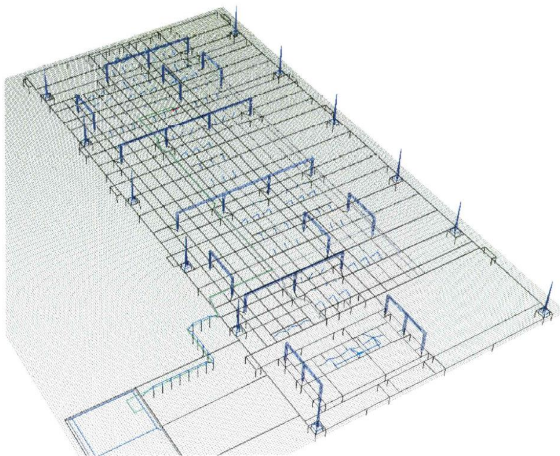
Рисунок 4- Трехмерный вид расчетной схемы ЗУ ОРУ 220 кВ в программе ОРУ- Проект
