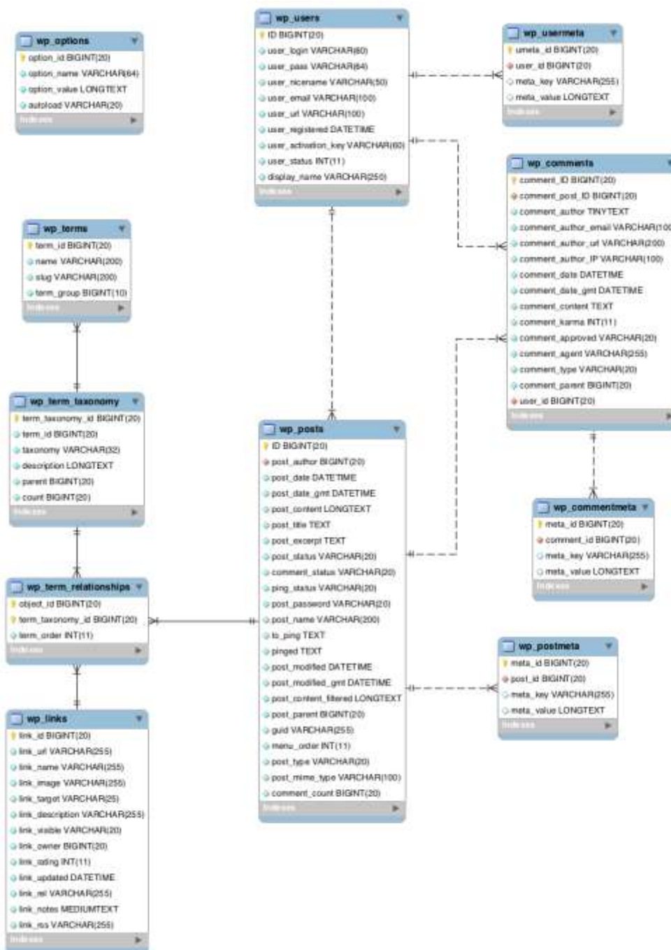
Рисунок 1 – Схема базы данных
