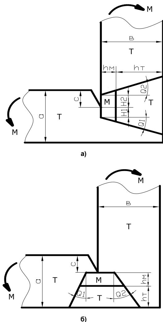
Рис. 1. Эскизы моделей сварных соединений: а – тип I; б – тип II
