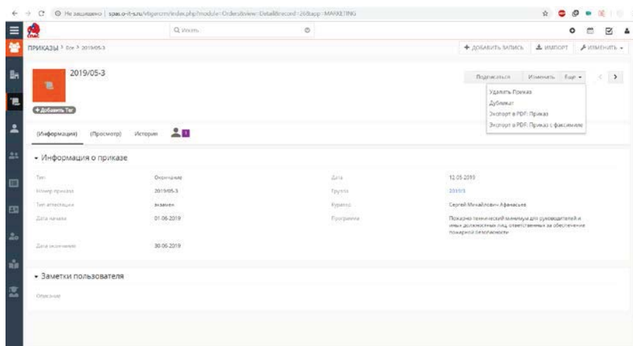
Рисунок 15 – Возможность экспорта в PDF «Приказ»
