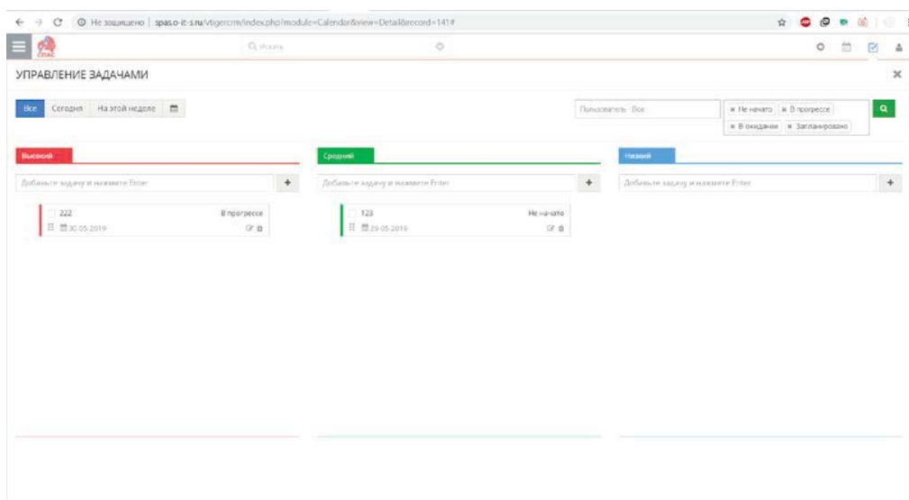
Рисунок 20 – Менеджер задач
