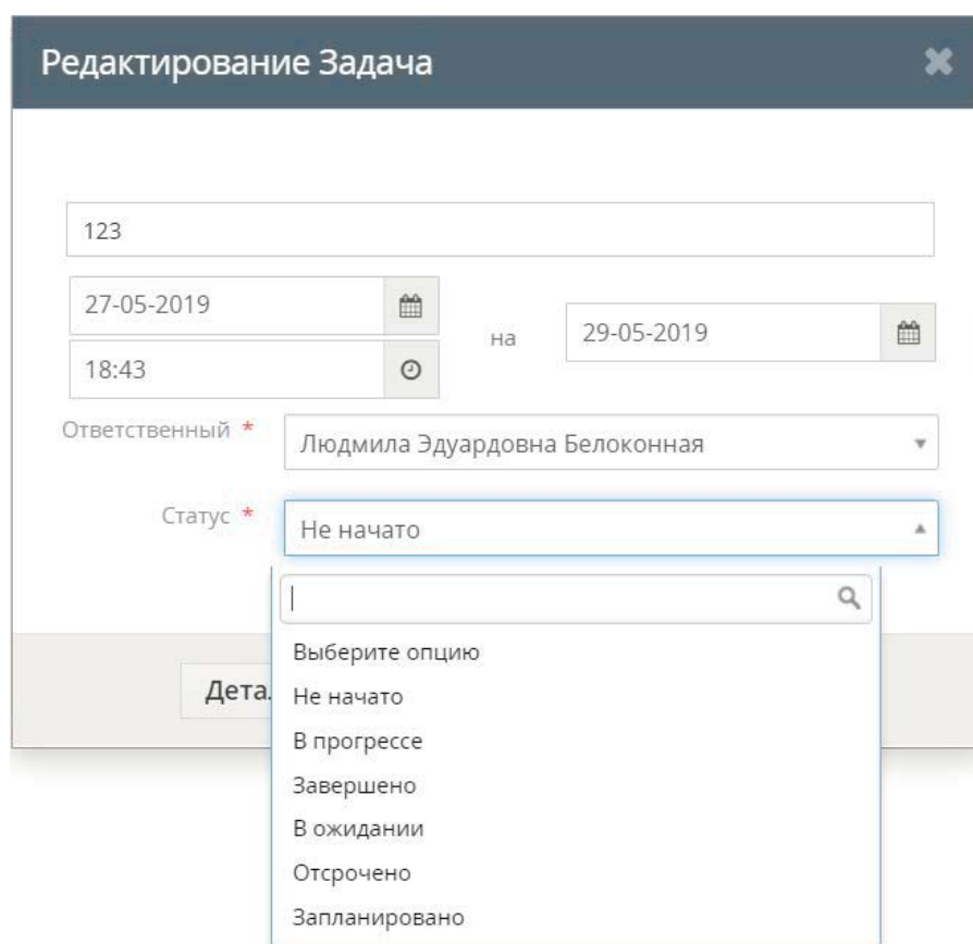
Рисунок 21 – Создание задач
