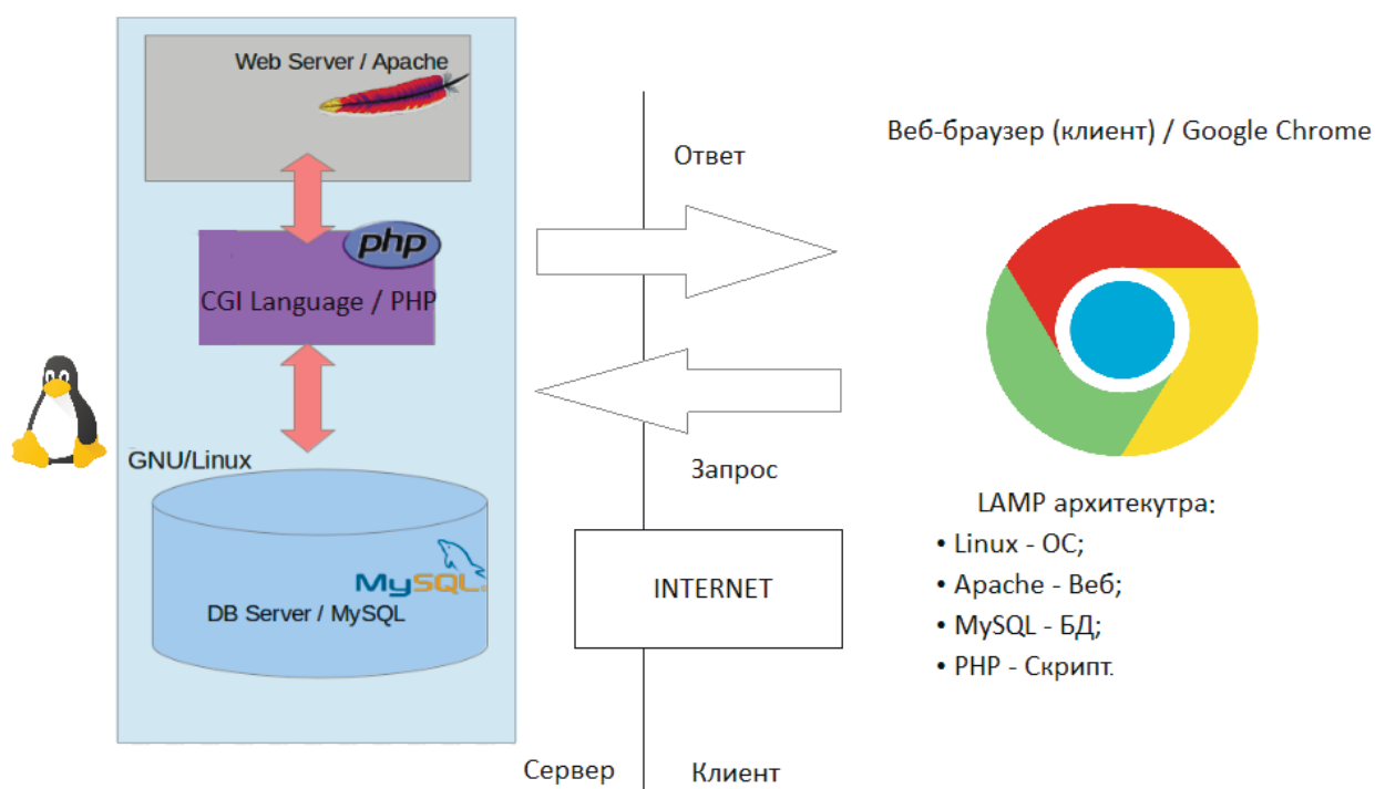
Рисунок 6 – Архитектура системы
