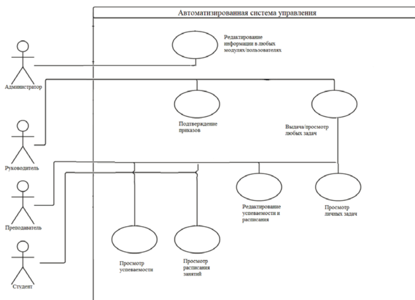
Рисунок 7 – Диаграмма прецедентов
