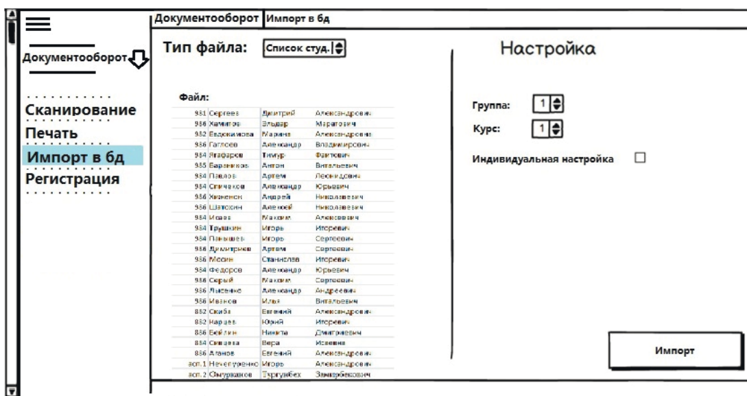
Рисунок 5 – Пример пользовательского интерфейса
