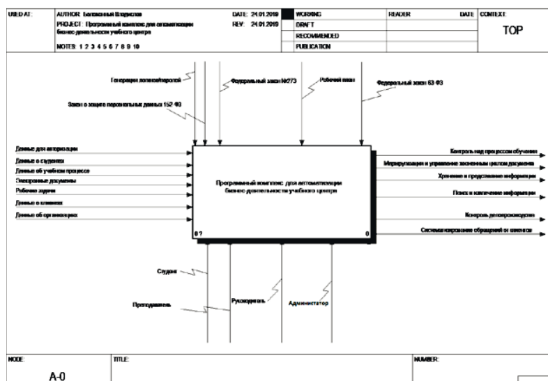
Рисунок 3 – Бизнес-процесс верхний уровень
