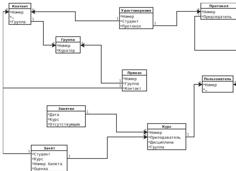
Рисунок 8 – Концептуальная схема базы данных
