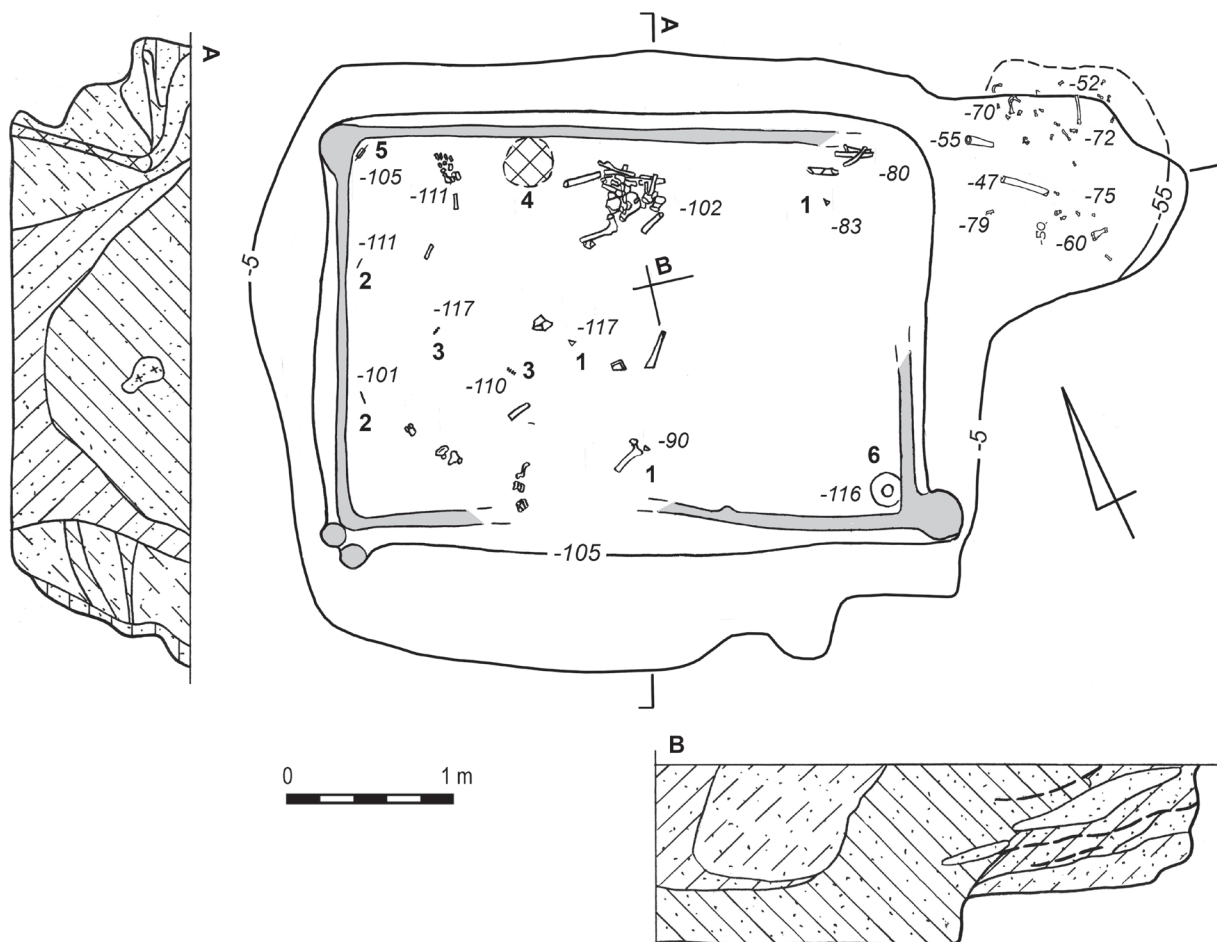
Рис. 2. Могильник Троицк-7. Курган 7. Могильная яма 1. План и разрезы. 1 — наконечник стрелы, 2 — бронзовые изделия, 3 — металлические украшения, 4 — пятно тлена, 5 — шило, 6 — сосуд
