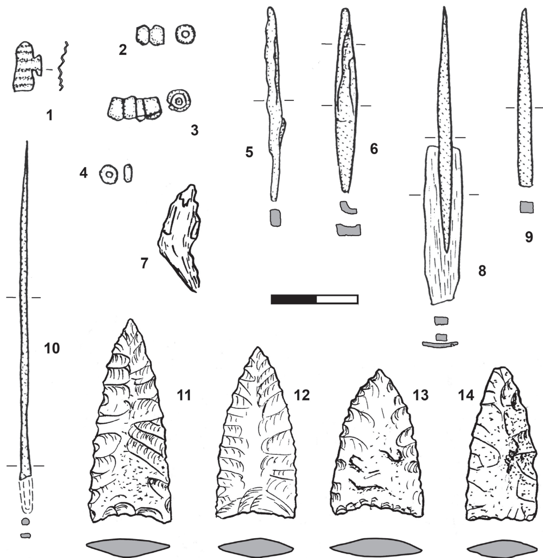
Рис. 3. Могильник Троицк-7. Курган 7. Могильная яма 1. Инвентарь. 1—3, 5—6, 8—10 — бронза; 4 — паста, 7 — кость, 11—14 — камень
