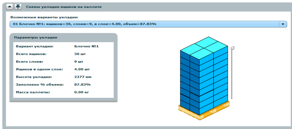
Рисунок 2.12 – Схема укладки ящиков на паллете
