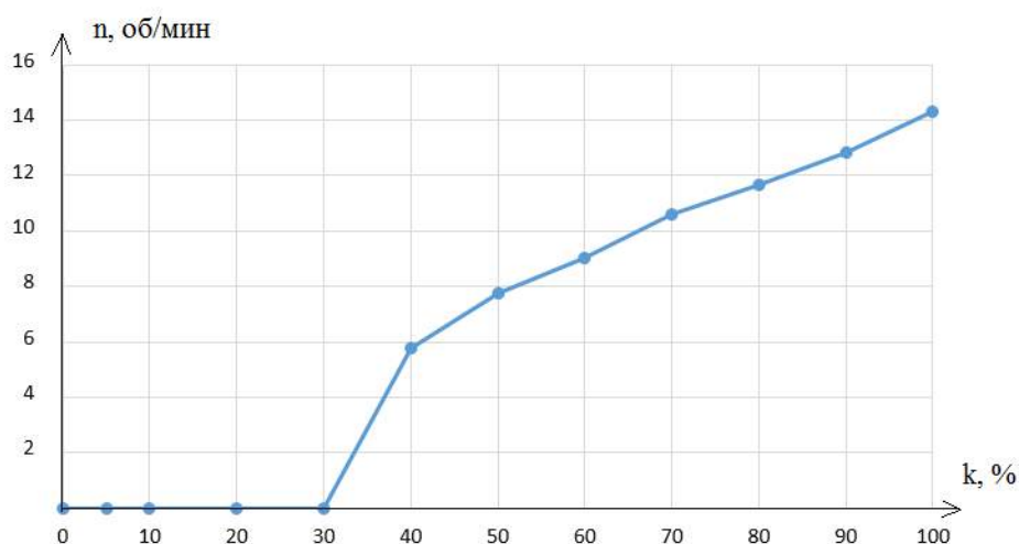
Рисунок 5.5 – Зависимость между коэффициентом заполнения ШИМ сигнала и частотой вращения ротора
