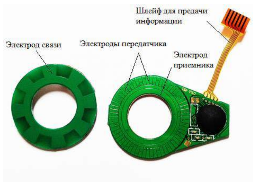
Рисунок 3.1 – Емкостная матрица
