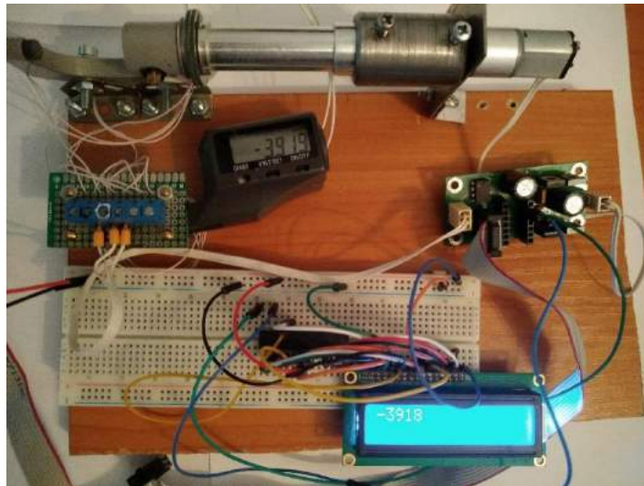
Рисунок 6.2 – Тестирование программы
