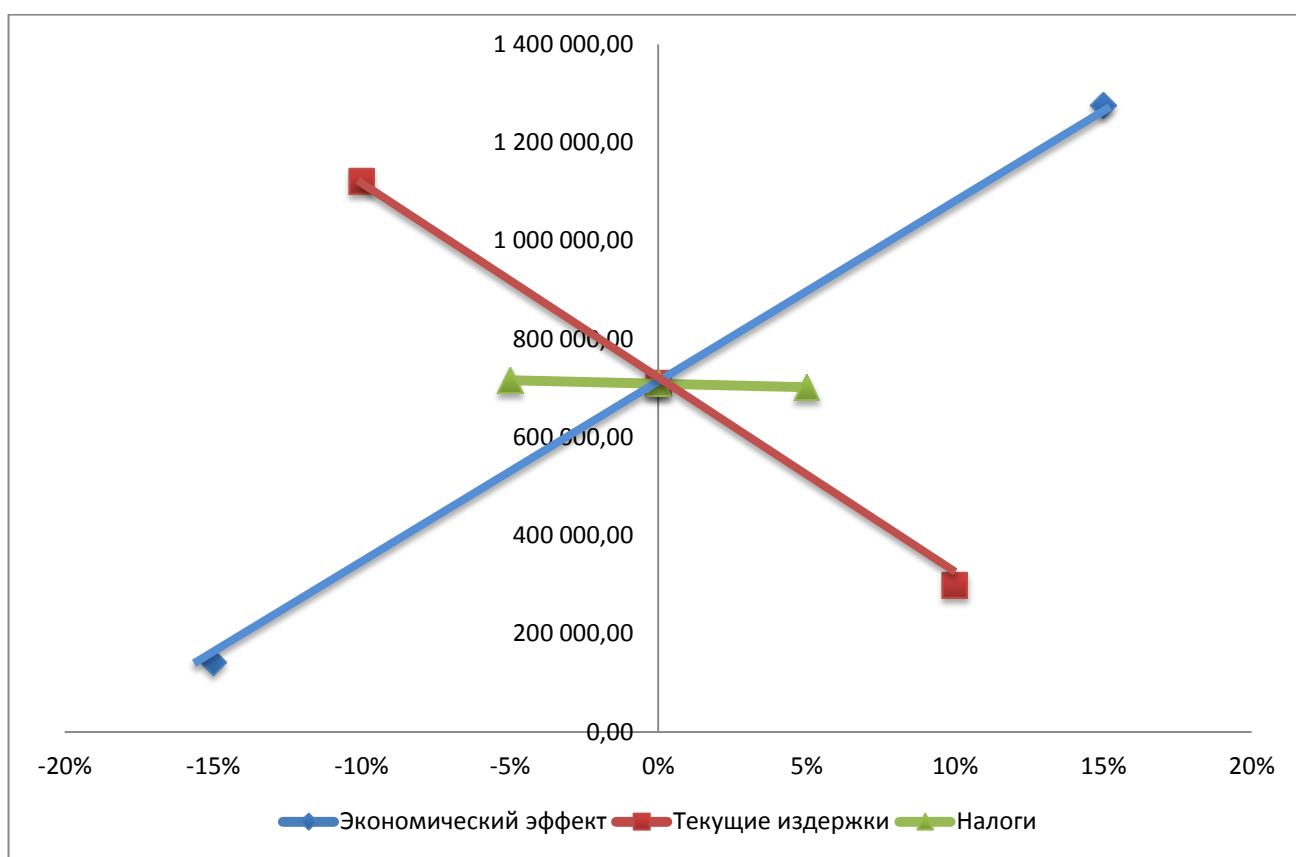
Рисунок 3.9 – Диаграмма «Паук»
