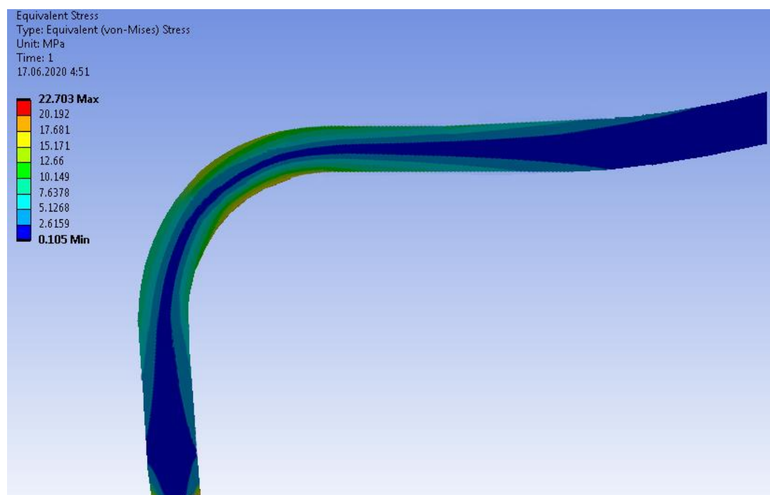
Рисунок 46 Эквивалентные напряжения в древесине
