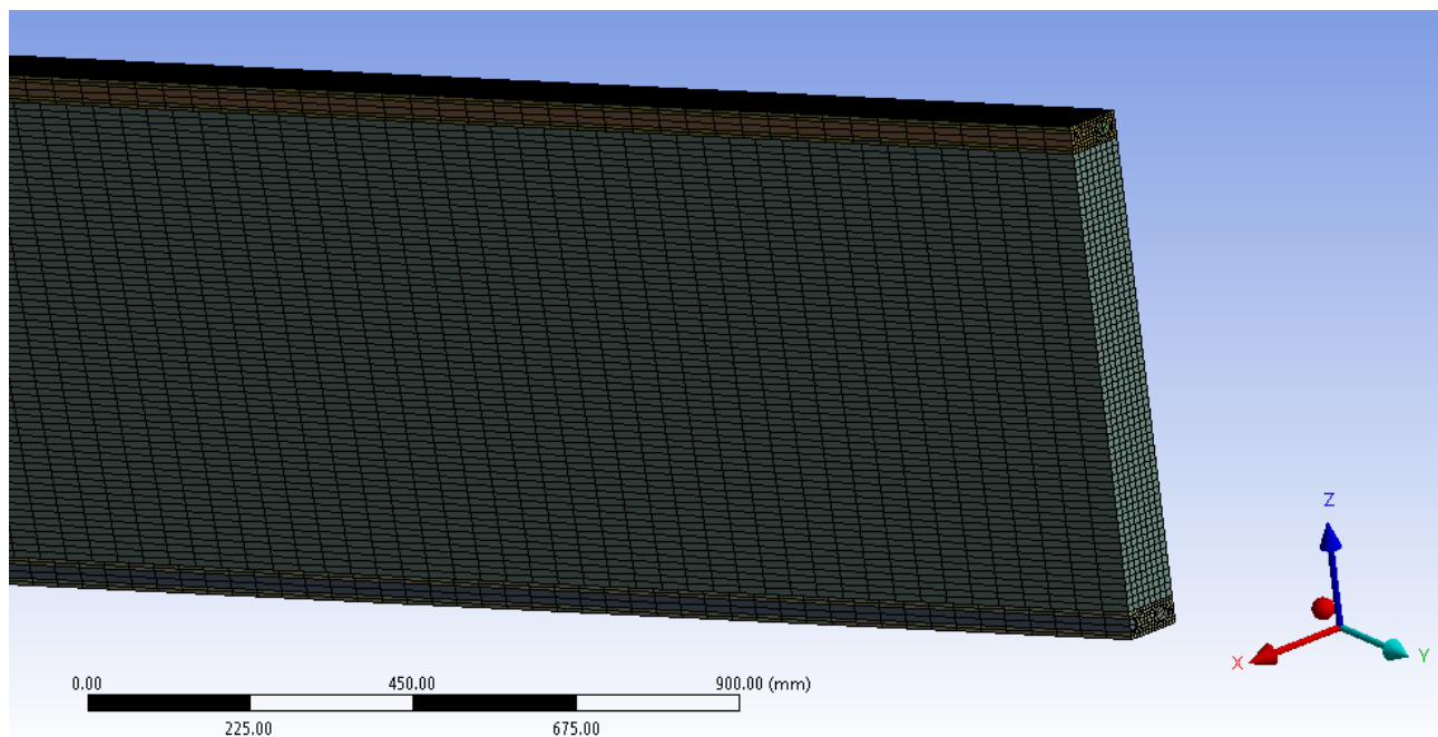
Рисунок 40 Элементы вблизи конькового узла
