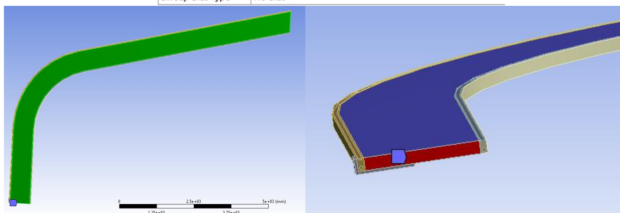
Рисунок 36 Параметры команды Sweep для центрального элемента древесины и выбранные для расчета элементы
