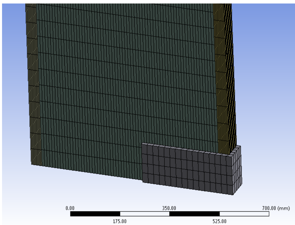
Рисунок 41 Опорный узел
