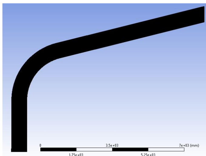
Рисунок 39 Общий вид конечноэлементной модели
