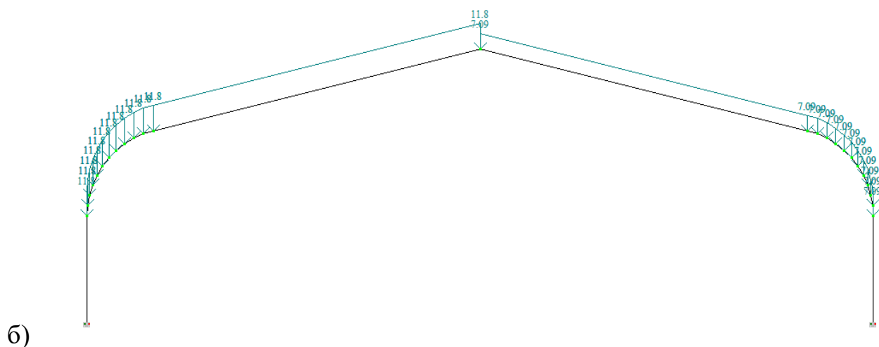
Рисунок 19. Снеговая нагрузка а) симметричная б) в отношении 1,25 : 0,75.
