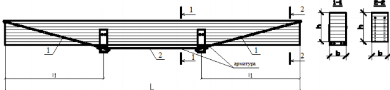
Рисунок 11. Армирование клееных деревянных балок
