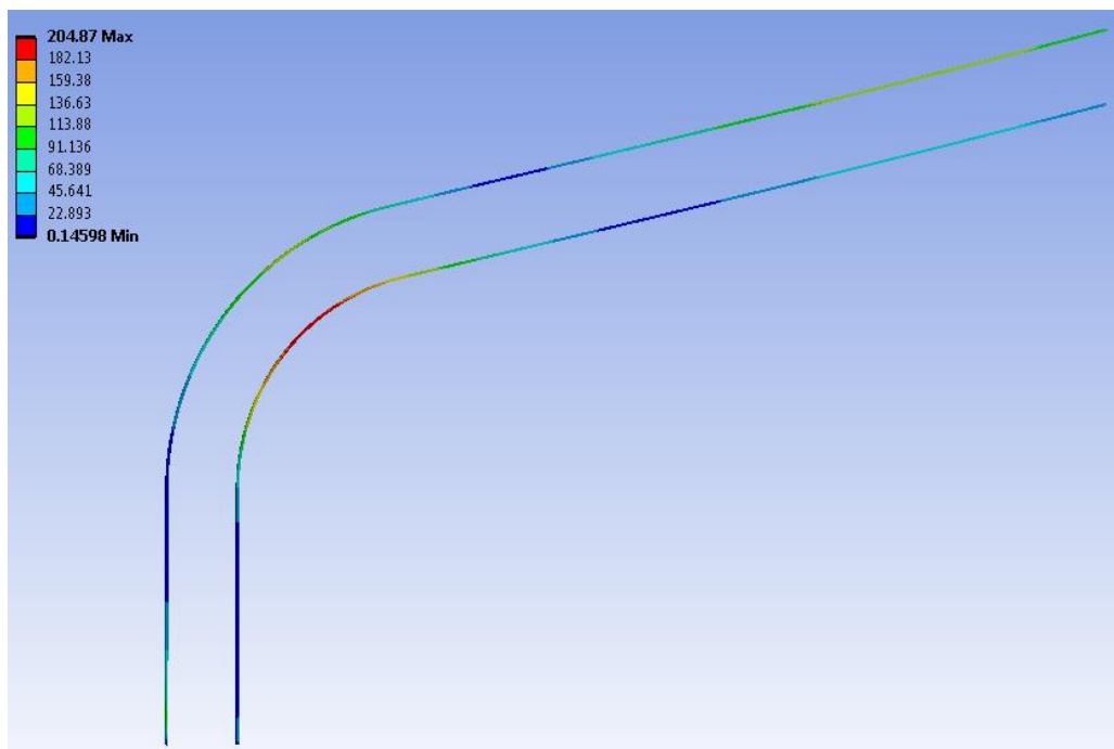
Рисунок 47 Эквивалентные напряжения в арматуре
