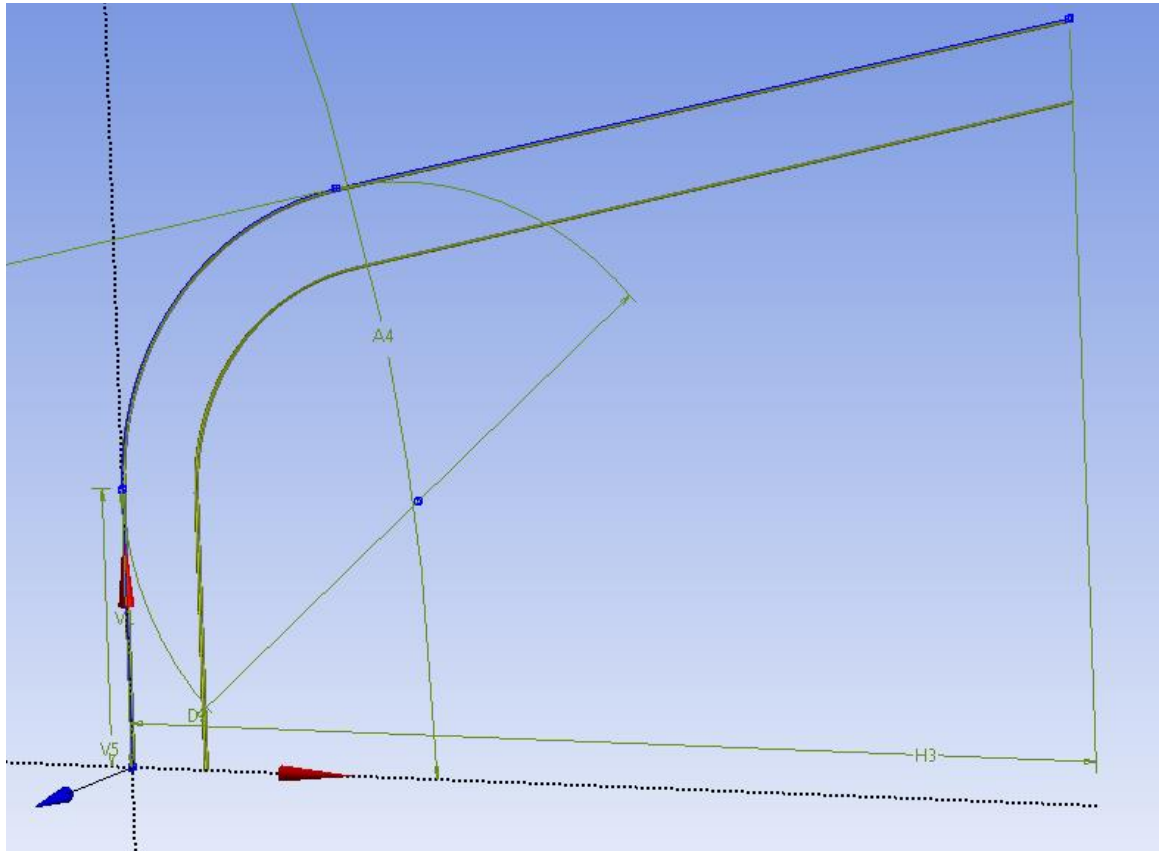
Рисунок 30 Созданные арматурные стержни
