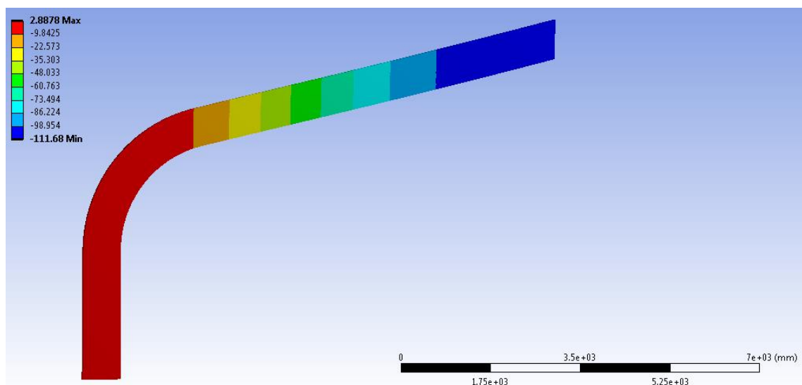
Рисунок 45 Деформации рамы вдоль оси Z
