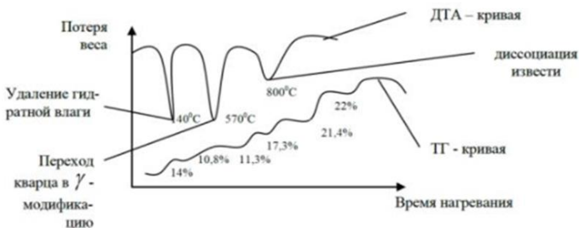
Рисунок 6 – Термограмма образца
