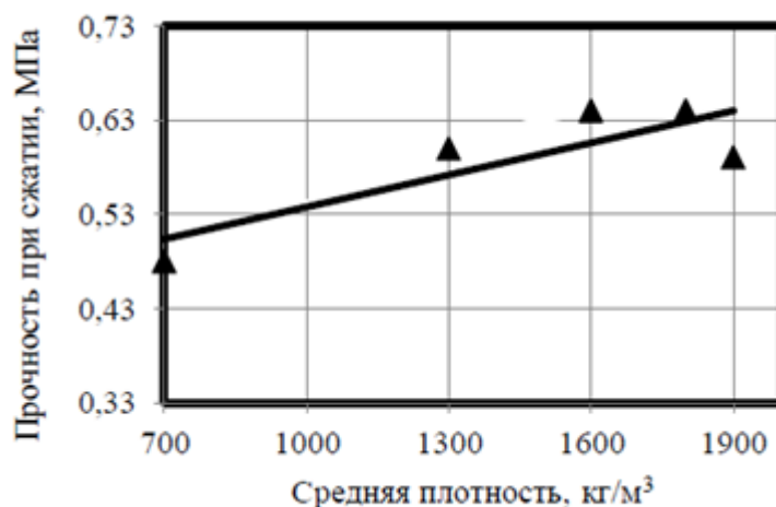
Рисунок 26 – Зависимость прочности при 10%-й линейной деформации перлитоволокнистого материала (30% волокна и 70% перлита, вспученного из фракции сырья 0,63–1,25 мм) от средней плотности породы
