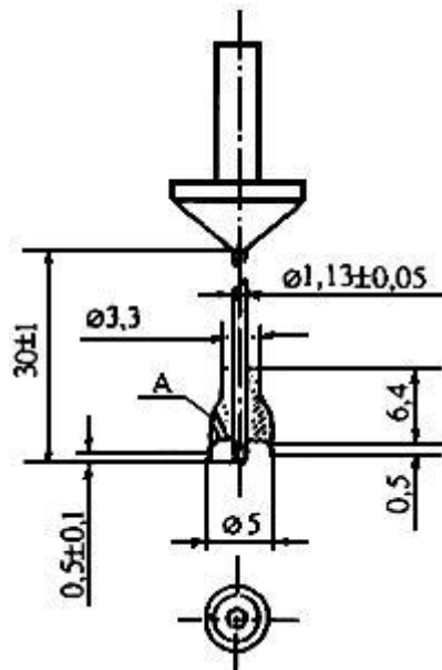
Рисунок 12 – Рабочая часть короткой иглы с кольцеобразной насадкой
