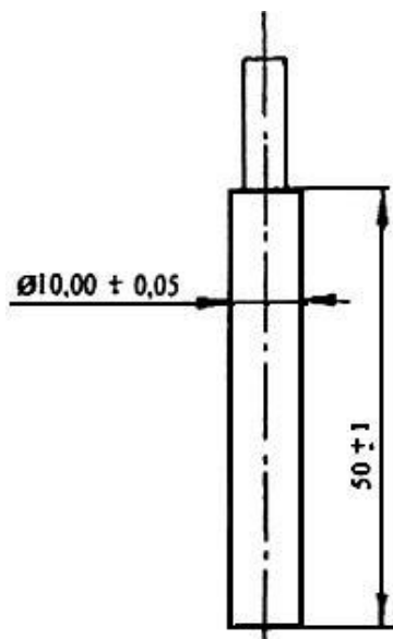
Рисунок 10 – Рабочая часть пестика
