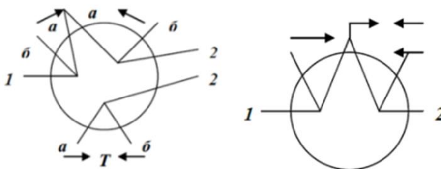
Рисунок 5 – Дифференциальный термопар
