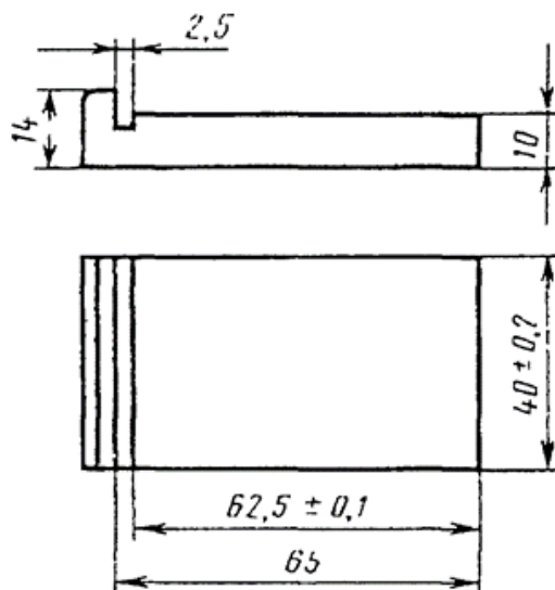
Рисунок 15 – Пластина
