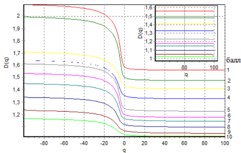
Рисунок 30 – Спектр обобщенных размерностей пластинчатого перлита
