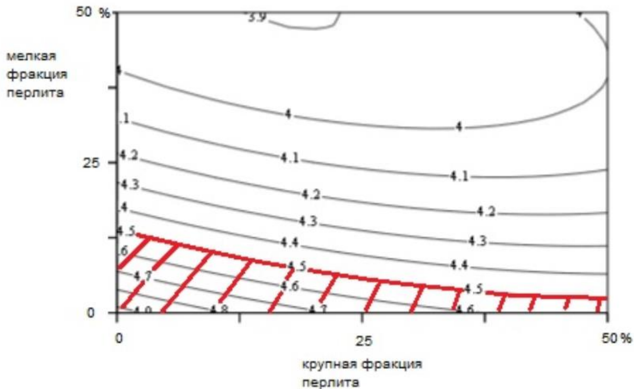
Рисунок 19 – КП+МП прочность на изгиб 28 сут
