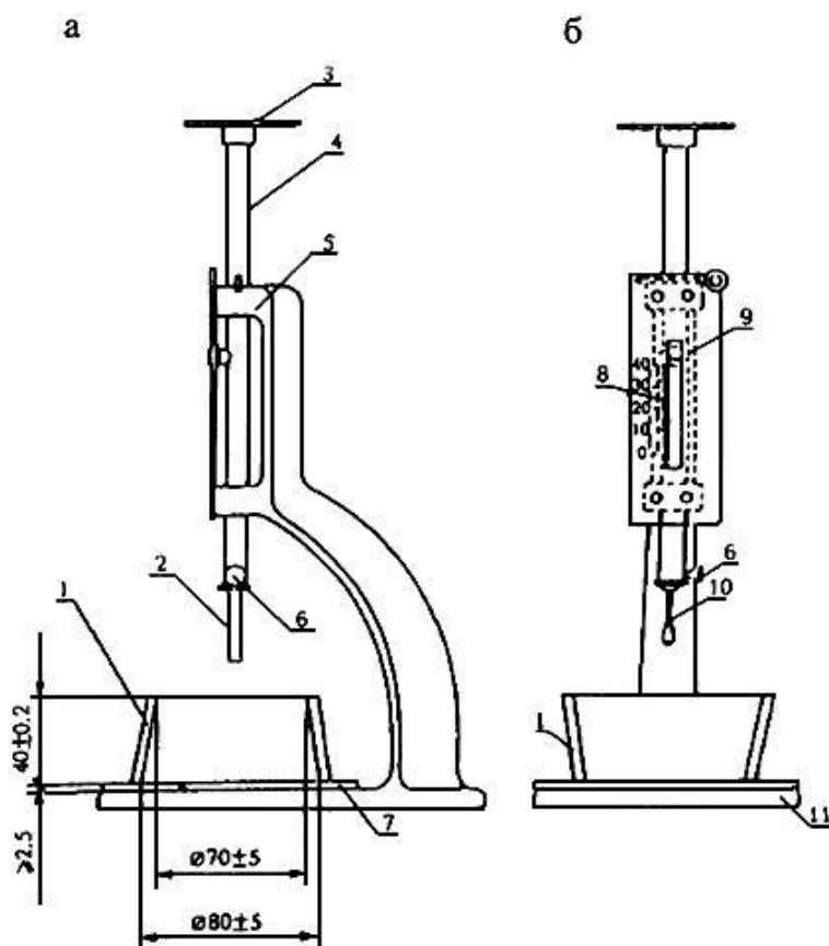
Рисунок 9 – Прибор Вика
