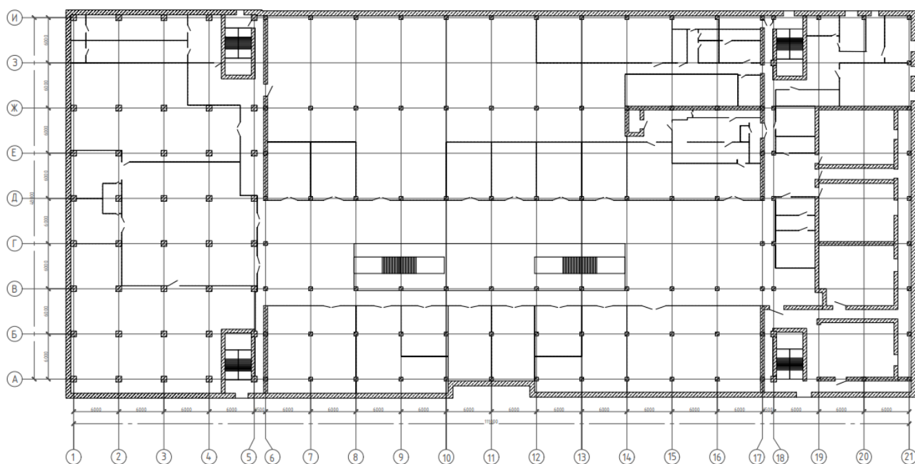
Рисунок В2 – Схема второго этажа
