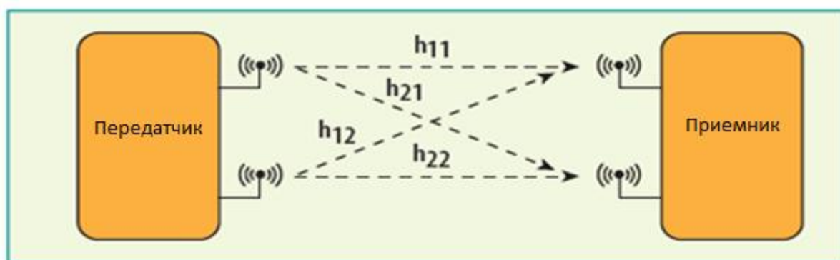
Рисунок 1 - Принцип работы системы MIMO 2x2
