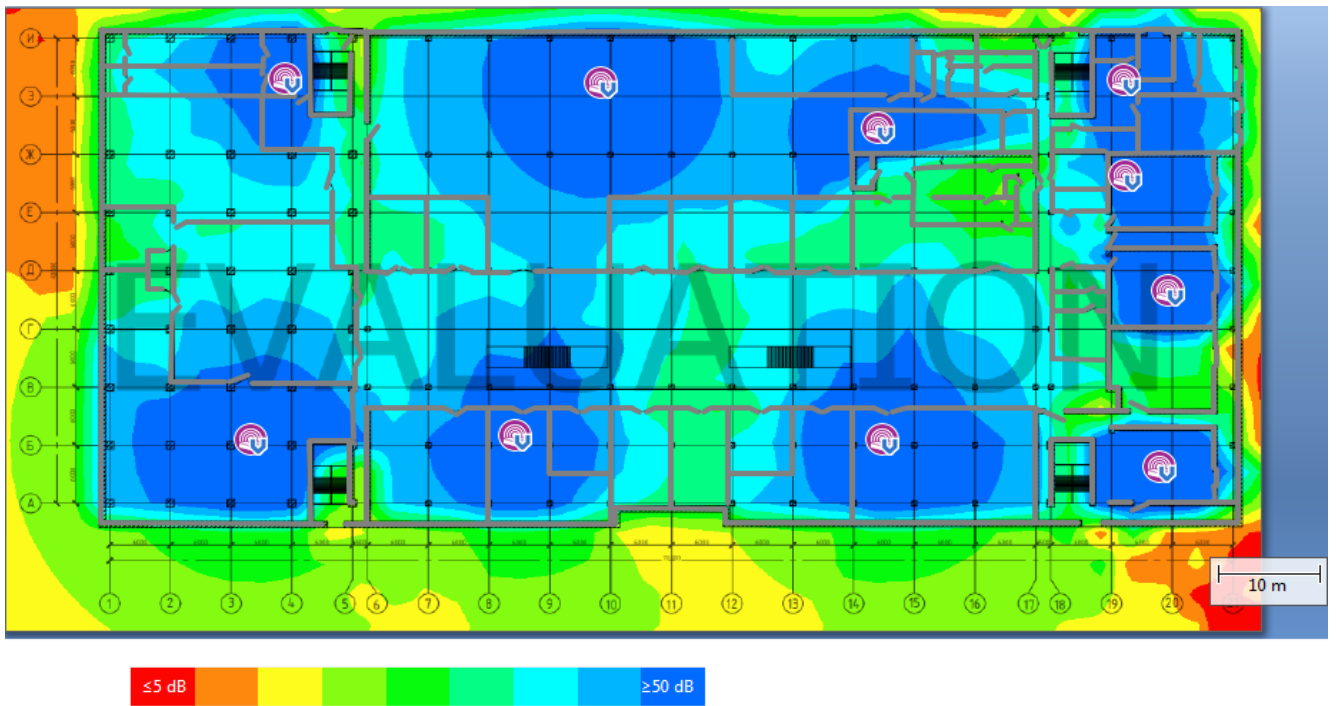
Рисунок 15 – Анализ отношения сигнал\шум
