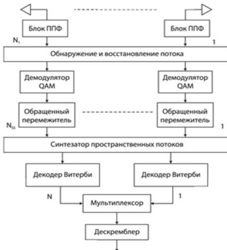
Рисунок 4 - Общая структура приемника MIMO-OFDM
