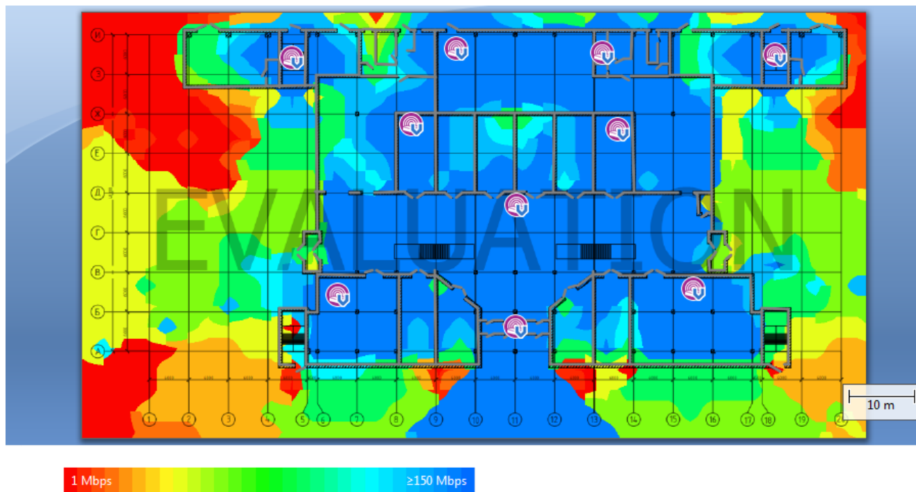
Рисунок 12 – Ожидаемая физическая скорость на первом этаже.
