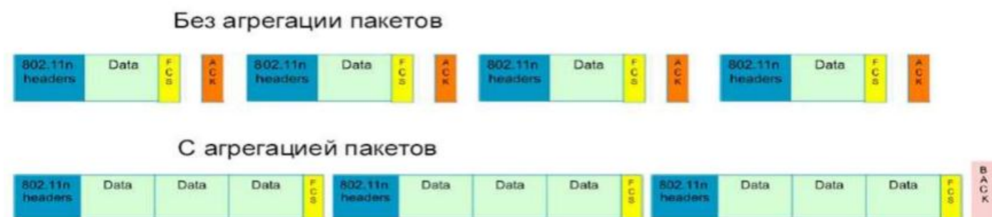
Рисунок 2 – Агрегация пакетов
