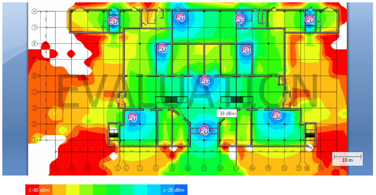
Рисунок 10 – Уровень сигнала на первом этаже
