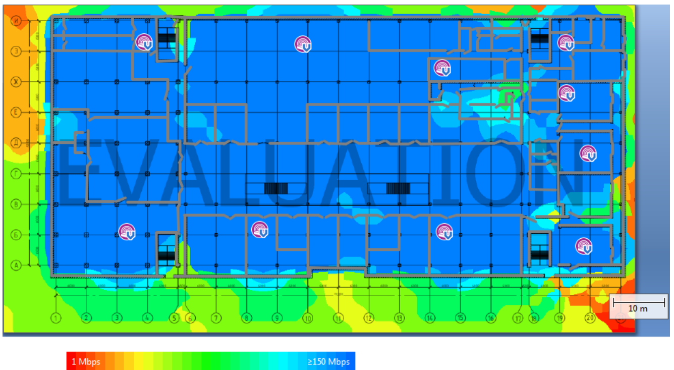
Рисунок 16 - Ожидаемая физическая скорость на втором этаже
