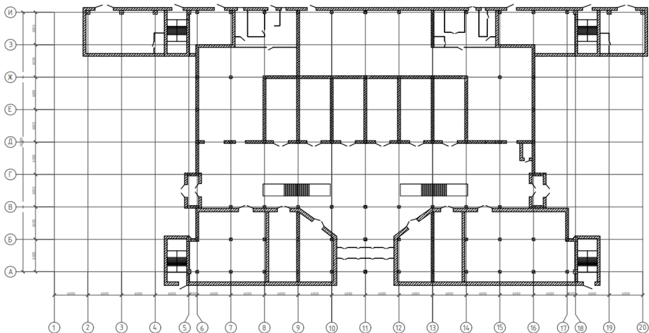
Рисунок 8 – Схема первого этажа торгового центра
