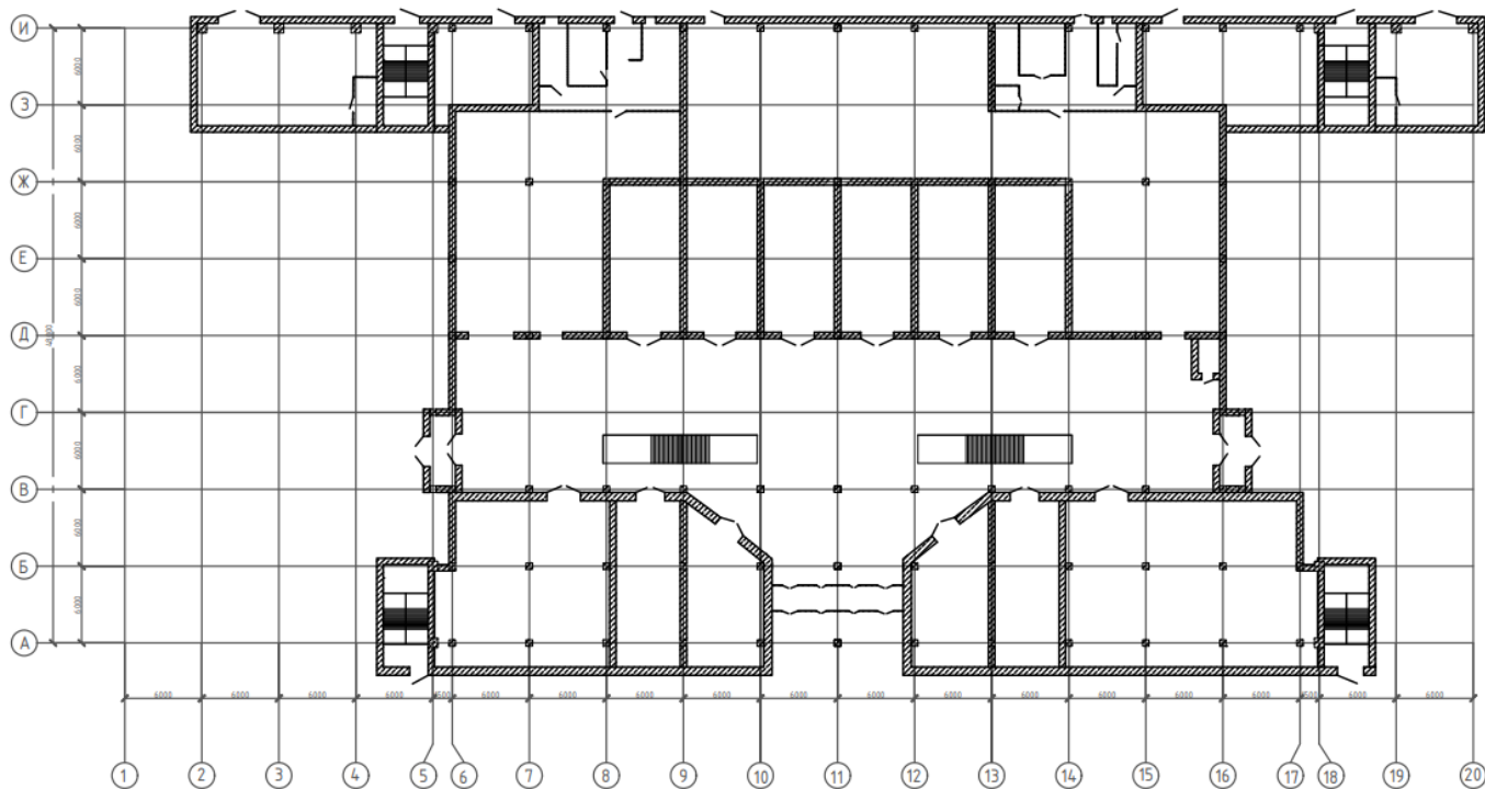
Рисунок В1 – Схема первого этажа
