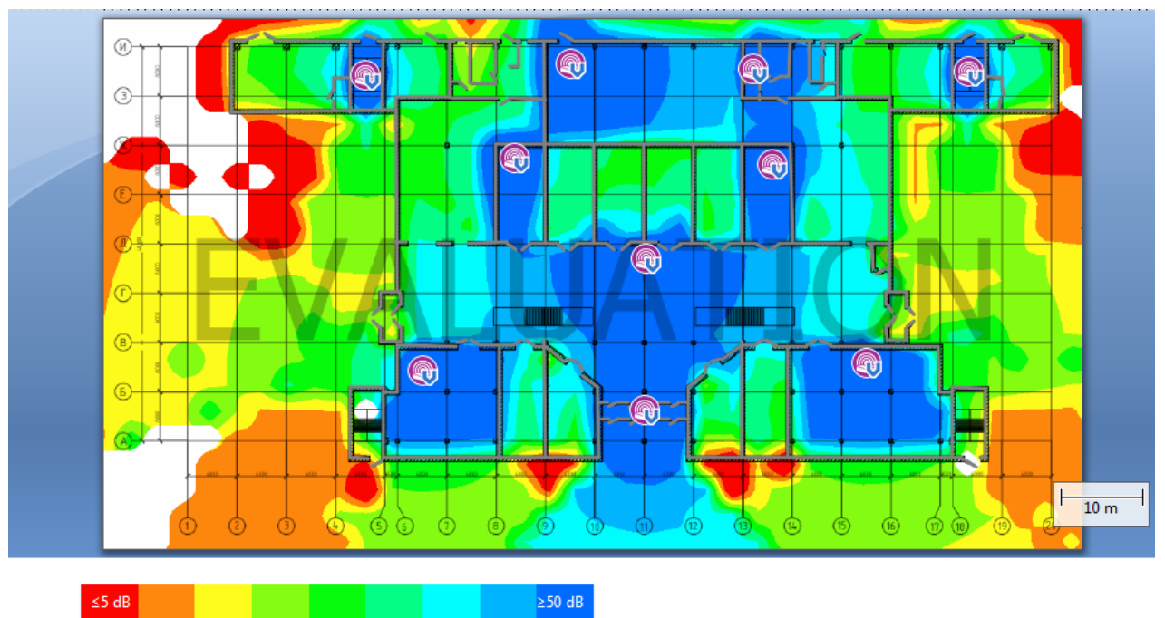
Рисунок 11 – Анализ отношения сигнал\шум
