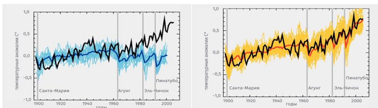
Рис. 1.2 График изменения климата за последние сто лет
