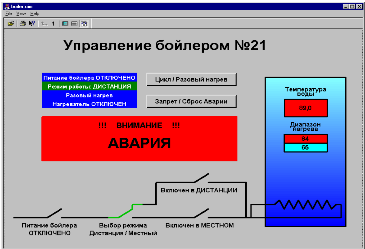
Рисунок 11 – Видеограмма аварийного режима отключения бойлер
