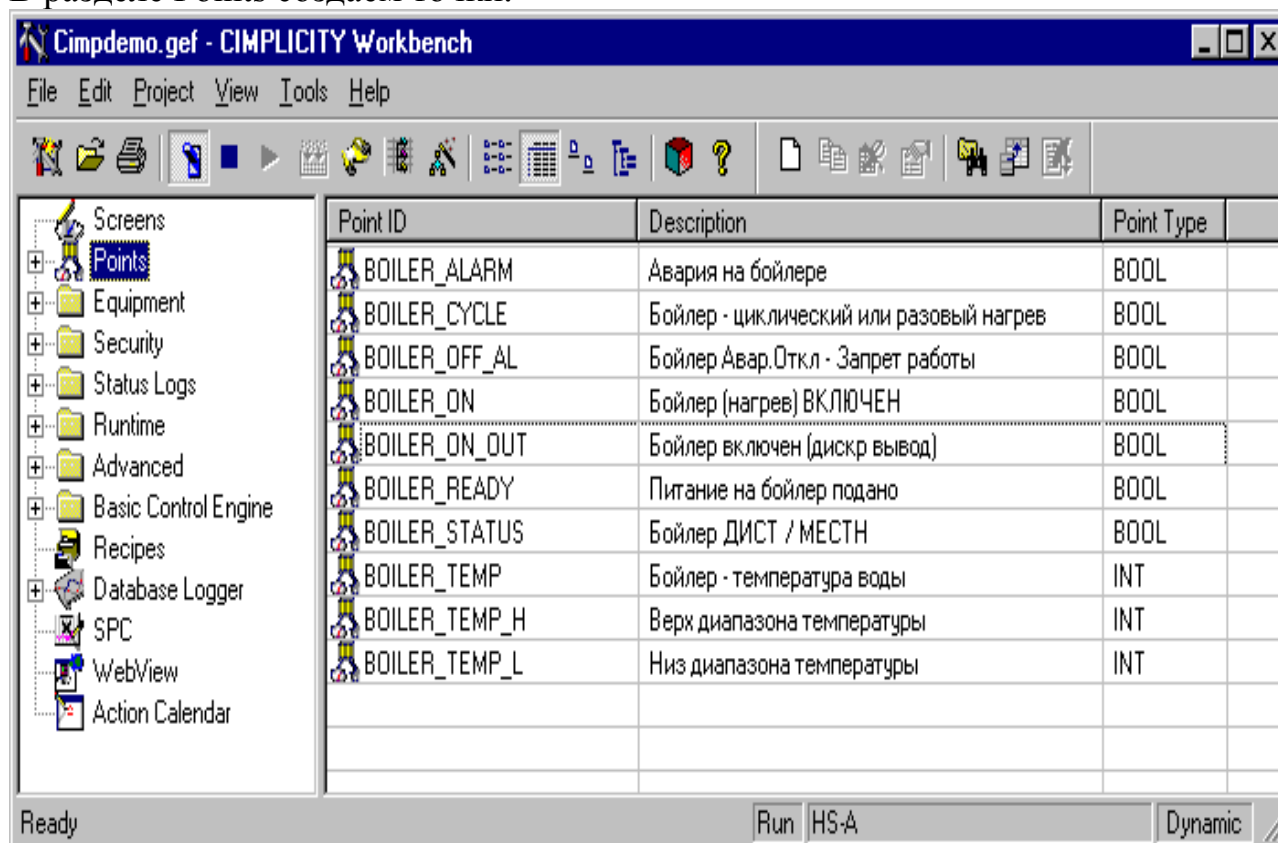
Рисунок 10 – Созданные контрольные точки для бойлера
