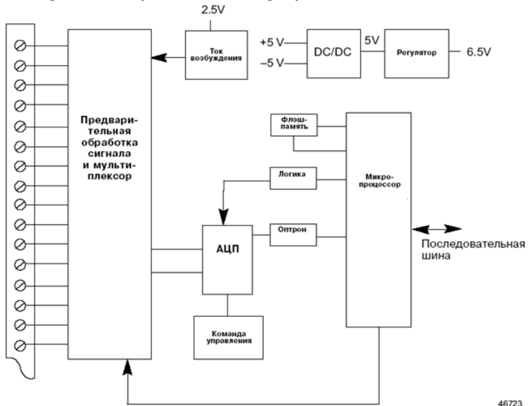
Рисунок 4 – Схема работы модуля
