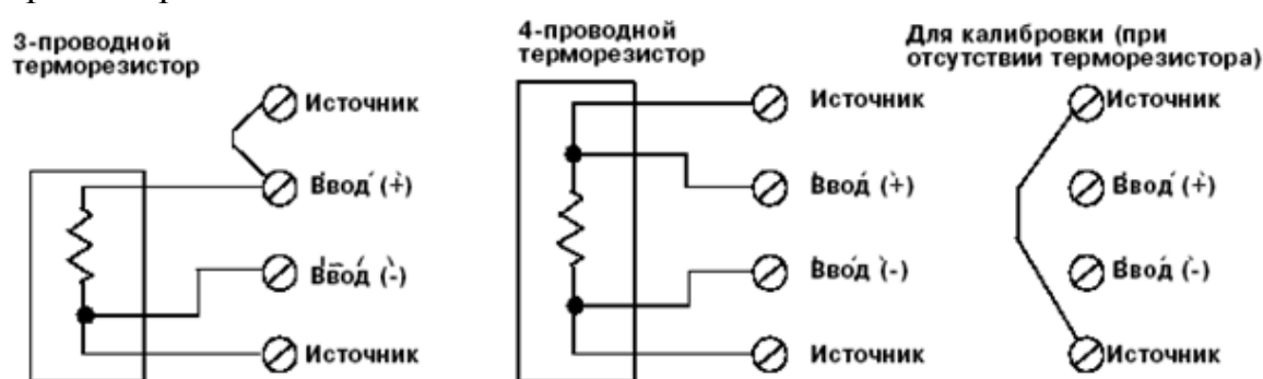
Рисунок 6 – Типы подключения терморезисторов
