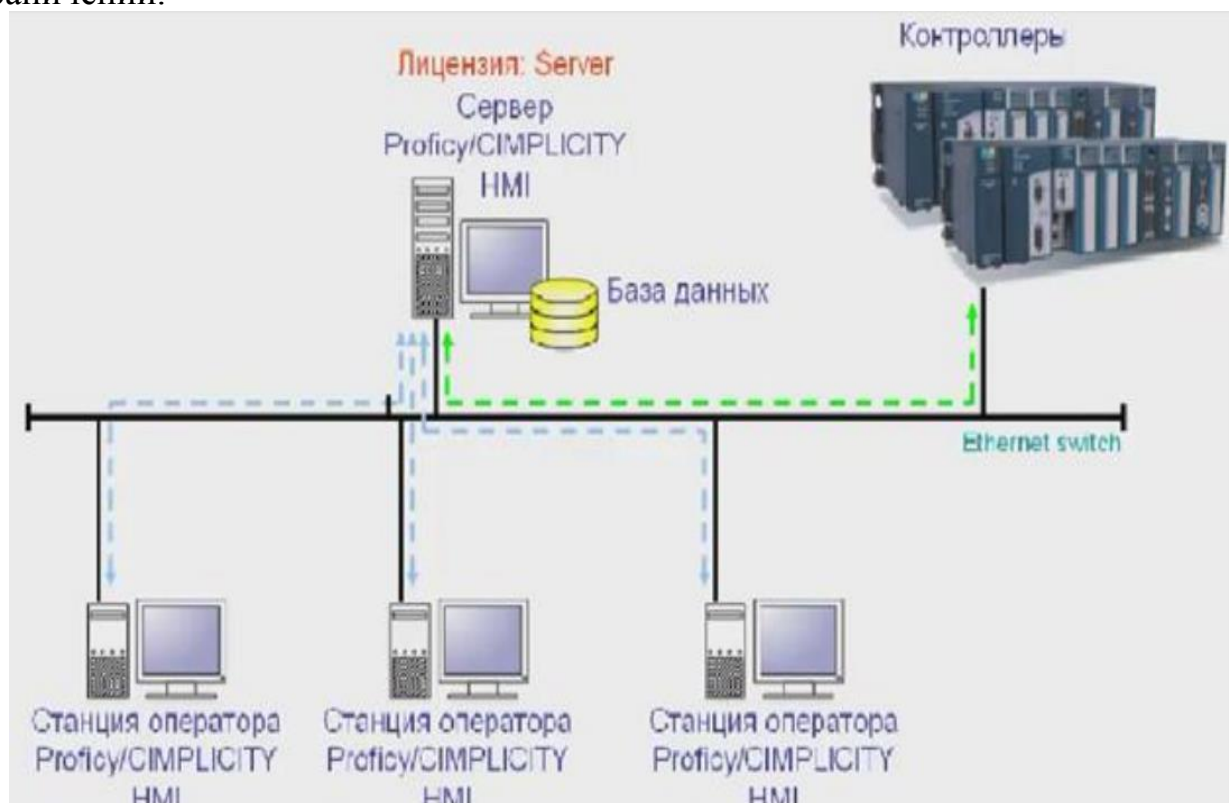
Рисунок 7 – Архитектура подсистемы АСУТП ХДМ УТС
