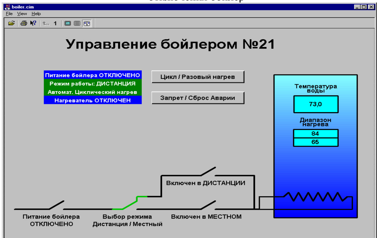
Рисунок 12 – Видеограмма отключенного от питания бойлера в дистанционном режиме с циклическим нагревом
