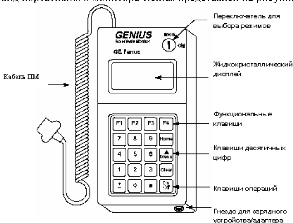
Рисунок 5 – Внешний вид портативного монитора Genius
