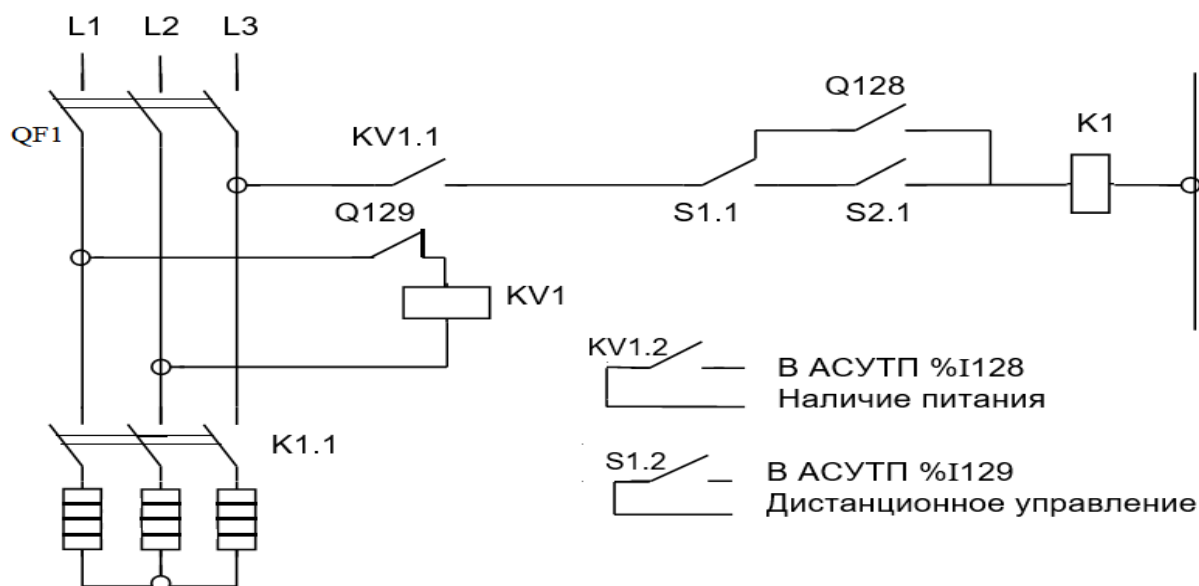
Рисунок 8 – Схема управления бойлером
