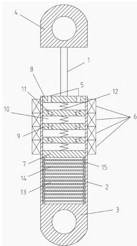
Рис. 2. Магнитореологический демпфер
