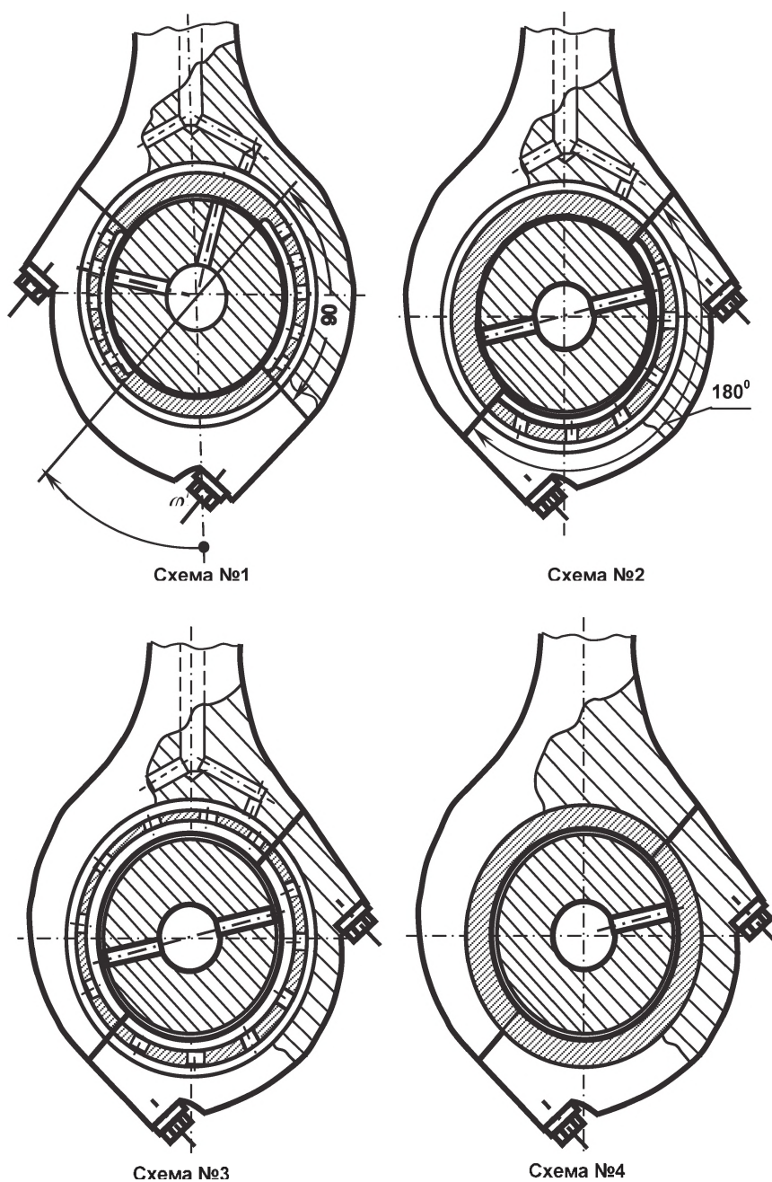
Рис. 2. Возможные схемы подачи смазки в шатунный подшипник двигателя ДМ-21
