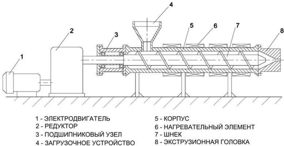
Рис. 1. Конструкция экструдера
