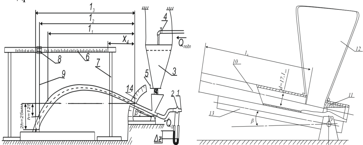
Рисунок 9 – Экспериментальной установки
