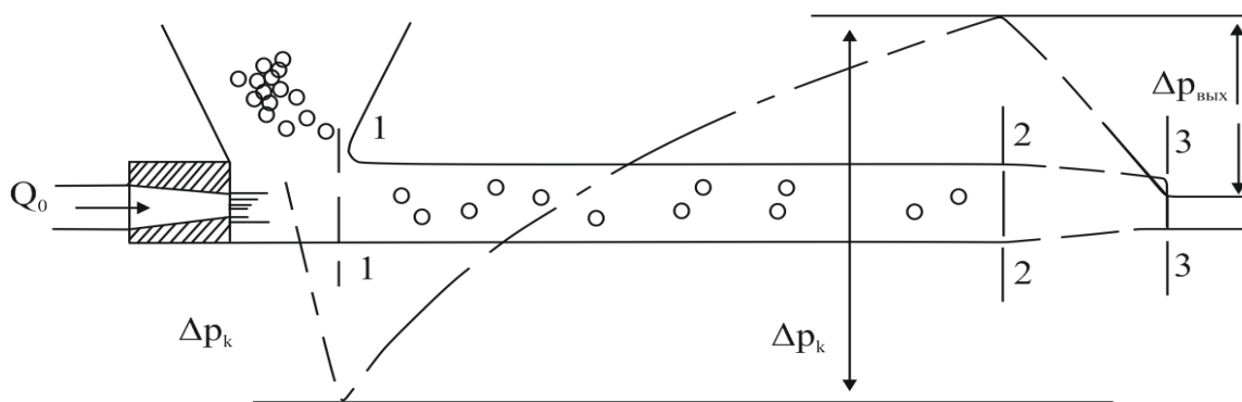
Рисунке – 5 Схема гидрометателя
