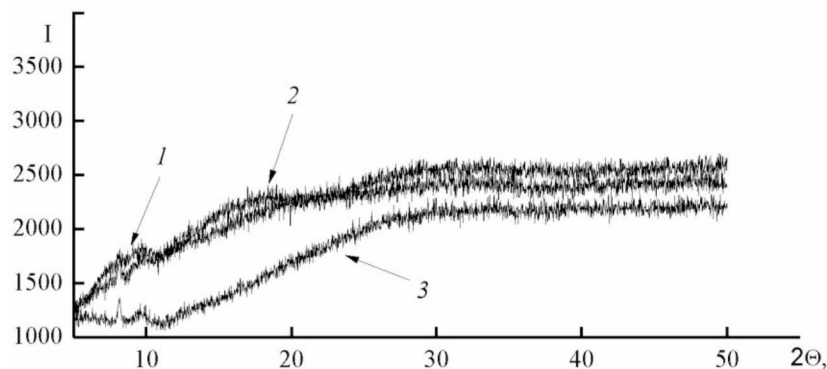
Рис. 2. Дифрактограммы аминиевых производных (1-гидроксиэтилиден)дифосфоната железа(II): 1 – \text{FeH}_2\text{L}\cdot\text{H}_2\text{NCH}_2\text{CH}_2\text{OH} , 2 – \text{FeH}_2\text{L}\cdot\text{H}_2\text{NC}(\text{CH}_2\text{OH})_3 , 3 – \text{FeH}_2\text{L}\cdot\text{H}_2\text{NCH}_2\text{CH}_2\text{OCH}_2\text{CH}_2\text{OCH}_2\text{CH}_2\text{NH}_2
