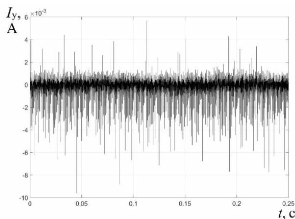
Рис. 3. Ток утечки при 1 кГц за 0,25 с ( U_{test} = 15 В)
