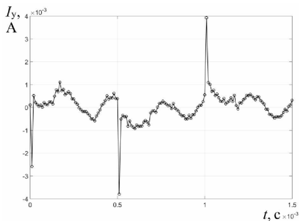
Рис. 4. Ток утечки при 1 кГц за 1,5 \cdot 10^{-3} с ( U_{test} = 15 В)
