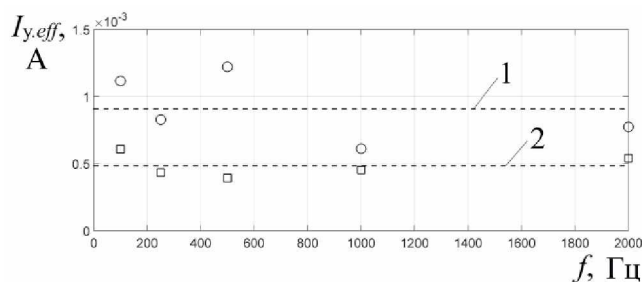
Рис. 6. Зависимости действующего значения тока утечки от частоты при двух амплитудах приложенного напряжения. Обозначено: \circ – 15 В; \square – 7,5 В; усредненные значения: 1 – 15 В; 2 – 7,5 В
