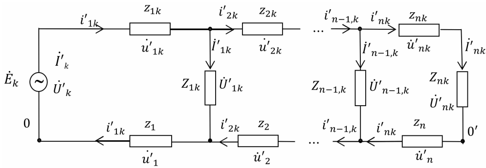
Рис. 2. Структура k -й подсистемы распределительной сети
