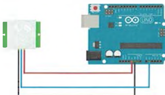
Рисунок 2.3 – Подключение HC-SR501 к Arduino Uno
