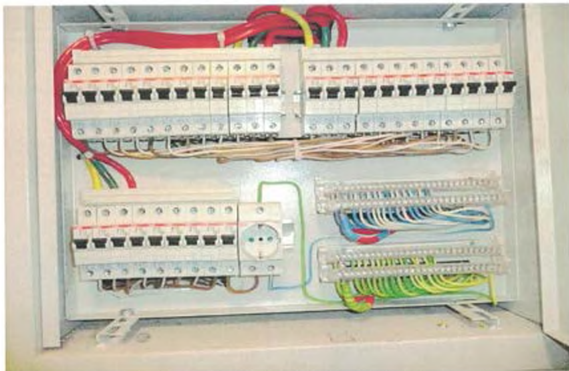
Рисунок 1.4 – Шкаф управления электрическими приборами
