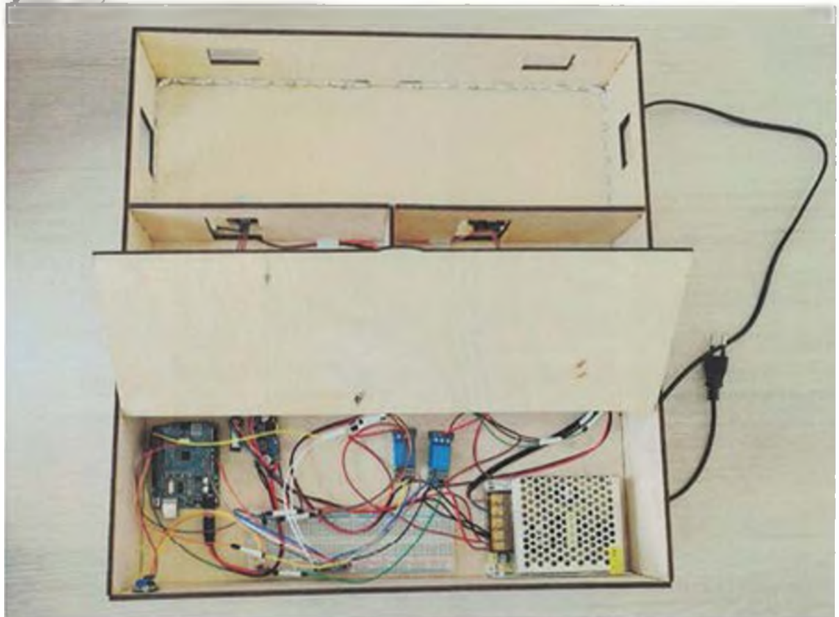
Рисунок 3.2 – Макет квартиры
