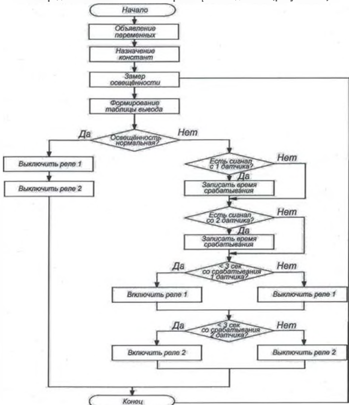
Рисунок 3.1 – Блок-схема алгоритма работы
