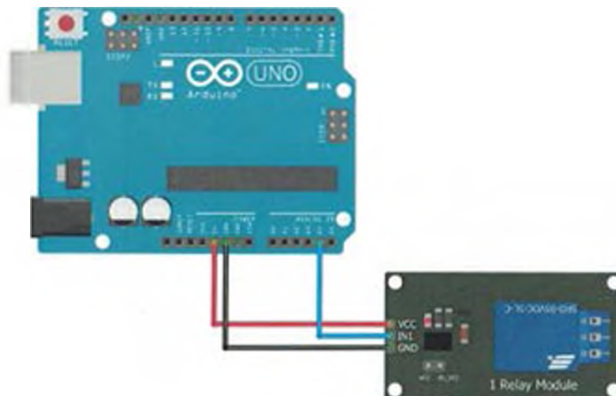
Рисунок 2.5 - Подключение реле к Arduino
