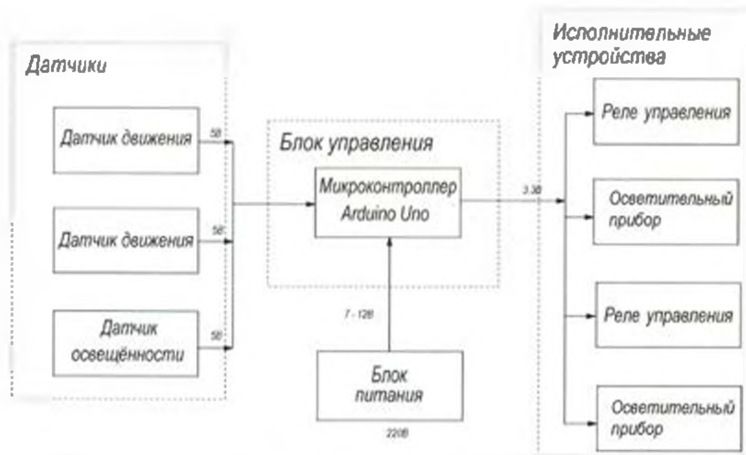
Рисунок 1.10 – Структурная схема системы освещения умного дома
