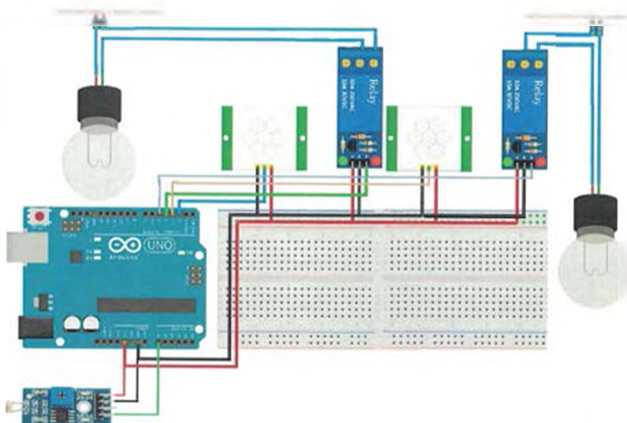
Рисунок 2.7 – Подключение системы управления
