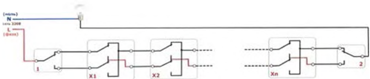
Рисунок 1.7 – Схема управления с освещением с 4 мест и более
