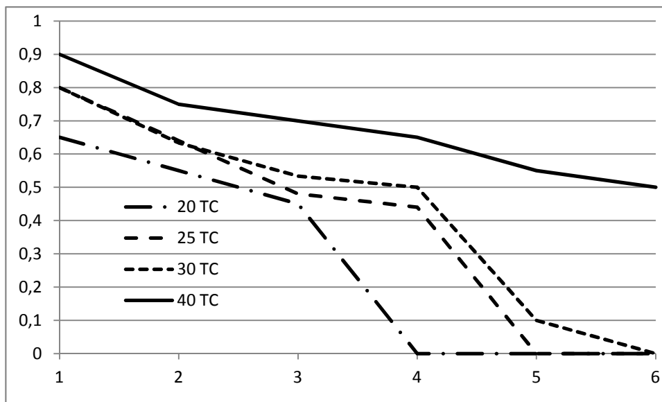
Рис. 5. Процент ТС, находящийся в резерве на момент окончания моделирования, в зависимости от общего количества ТС и продолжительности моделирования (мес.) Fig. 5. Percentage of vehicles in reserve at the end of the simulation, depending on the total number of vehicles and the duration of the simulation (months)
