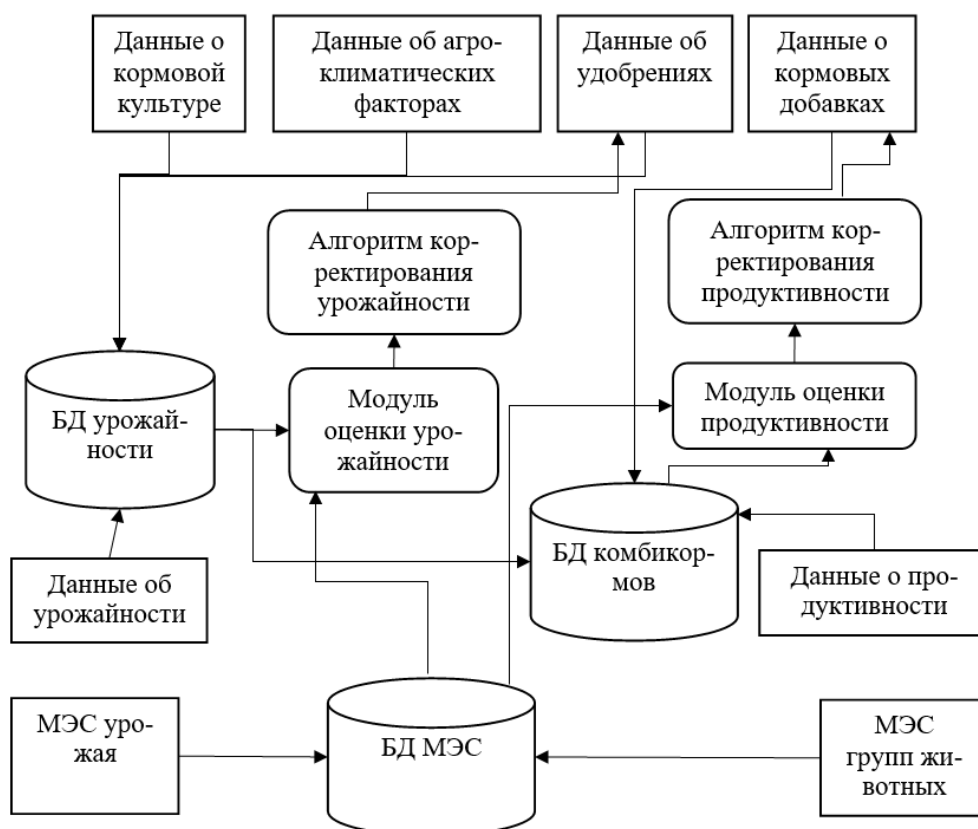
Рис. 2. Блок-схема СППР в области молочного животноводства
