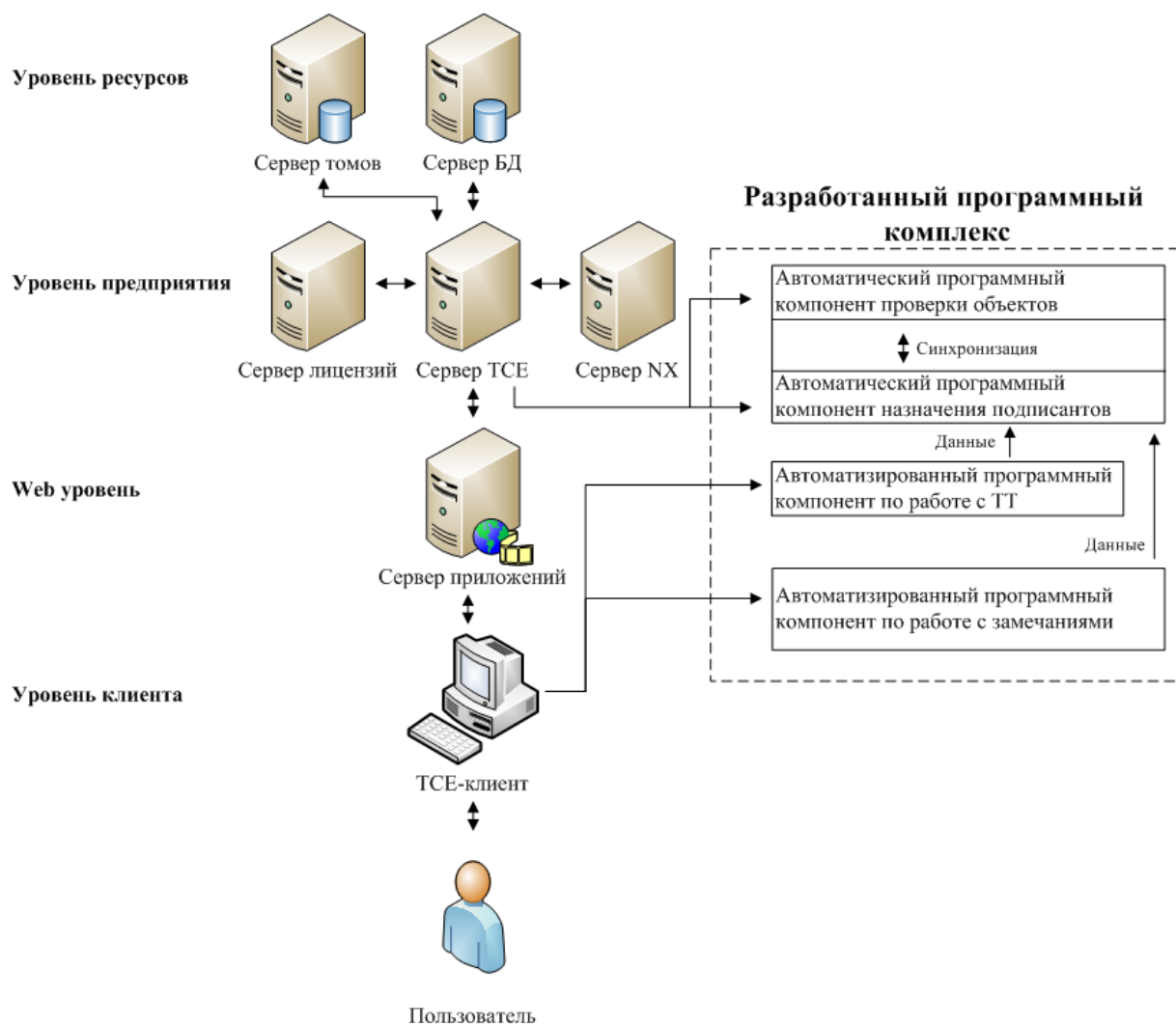
Рис. 5. Компоненты ПК в составе Teamcenter Fig. 5. Components of the software complex in architecture Teamcenter
