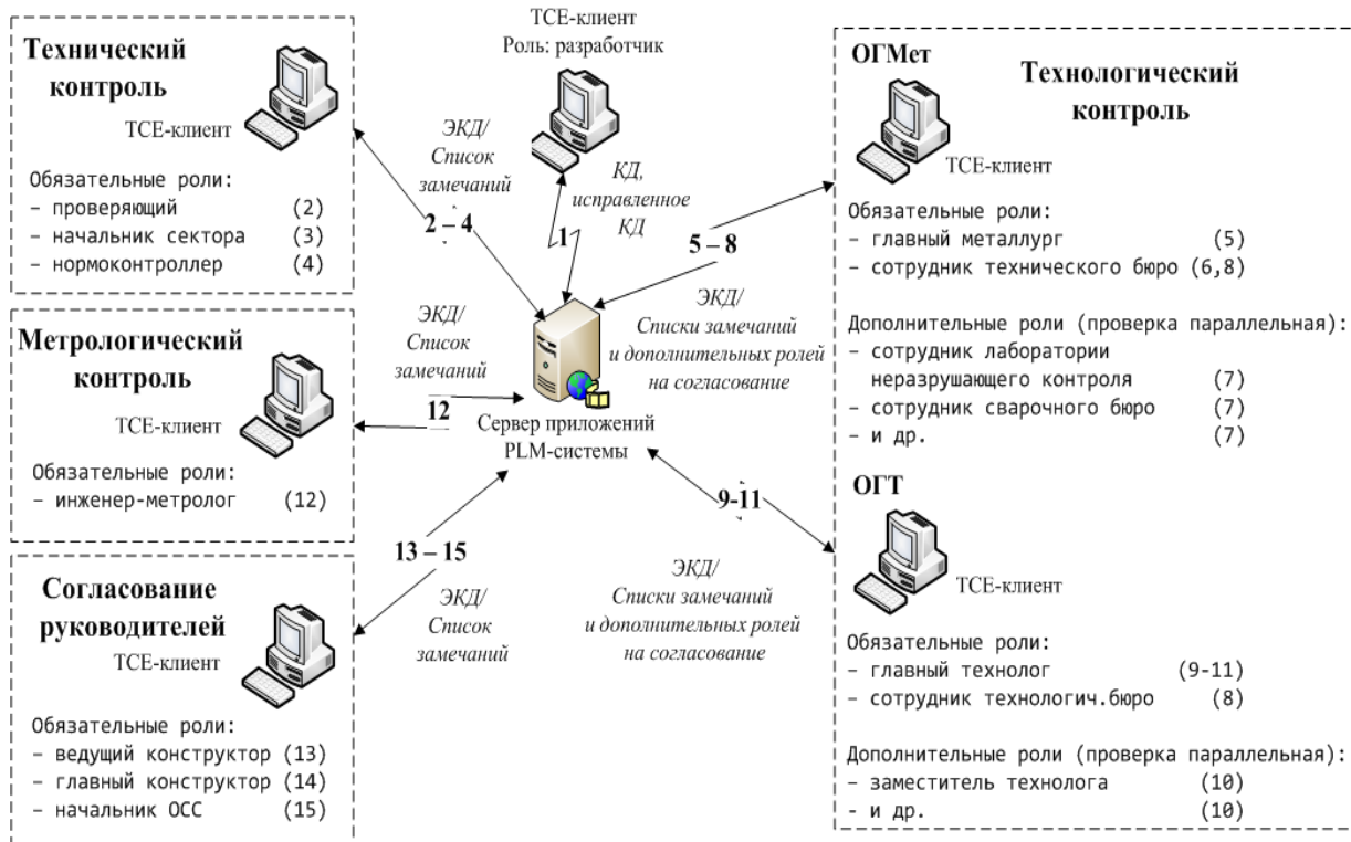
Рис. 3. Мнемосхема существующего бизнес-процесса в PLM-системе Fig. 3. Mnemonic diagram of an existing business process in a PLM-system
