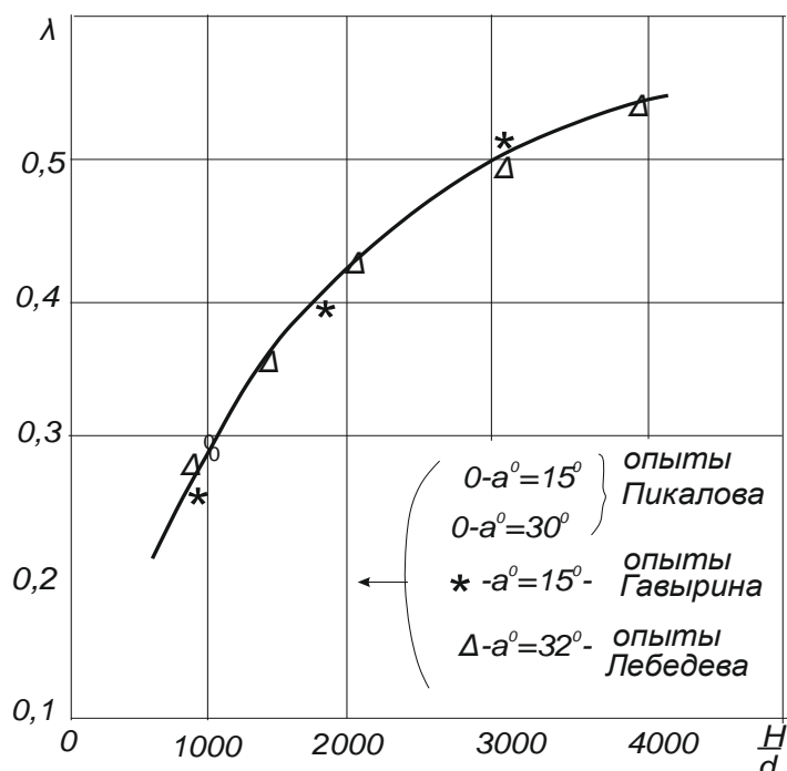
Рис. 3. Зависимость коэффициента трения от отношения напора к диаметру 4
