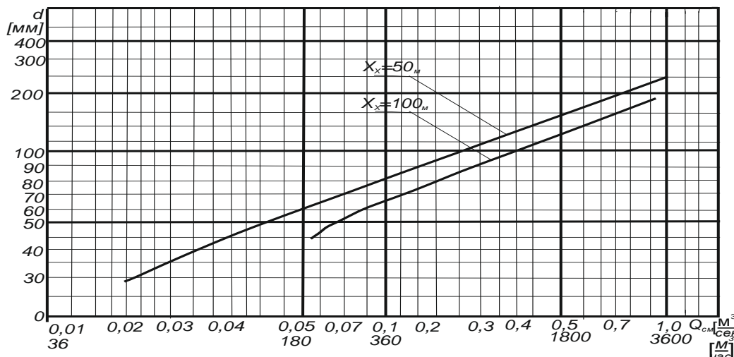
Рис. 4. Вспомогательный график к расчету диаметра рабочей камеры
