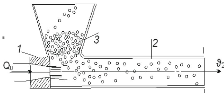
Рис. 1. Схема гидрометателя
