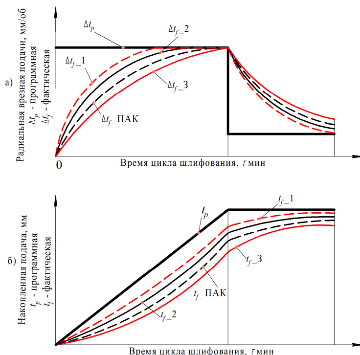
Рис. 3. Графики параметров двухступенчатого цикла круглого врезного шлифования вала с переменной податливостью по длине обрабатываемой поверхности: а – графики радиальной программной и фактической подачи; б – графики накопленных программной и фактической подач при двухступенчатом цикле шлифования
