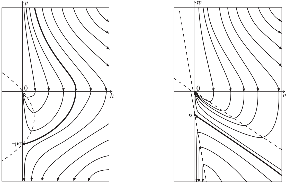
Фазовые портреты систем (13) и (14)
