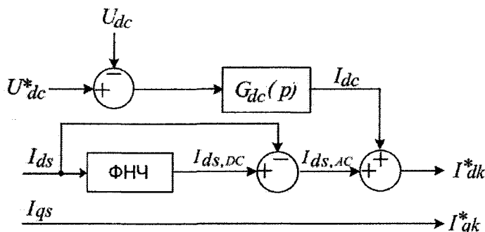
Рис. 6. Структурная схема блока определения опорных токов
