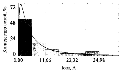
Рис. 5. Плотность вероятности логарифмически нормального распределения I_{OЗЗ} в городских электрических сетях
