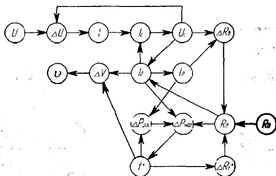
Рис. 14. Граф определения параметров разрушения фазного провода ВЛ
