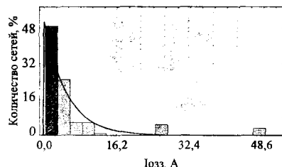
Рис. 6. Плотность вероятности экспоненциального распределения I_{OЗЗ} в сельских электрических сетях
