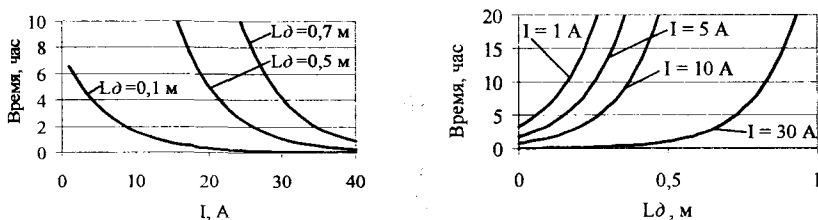
Рис. 12. Зависимость времени пережога проволоки наружного повива токоведущей части провода АС-70 от параметров дуги
