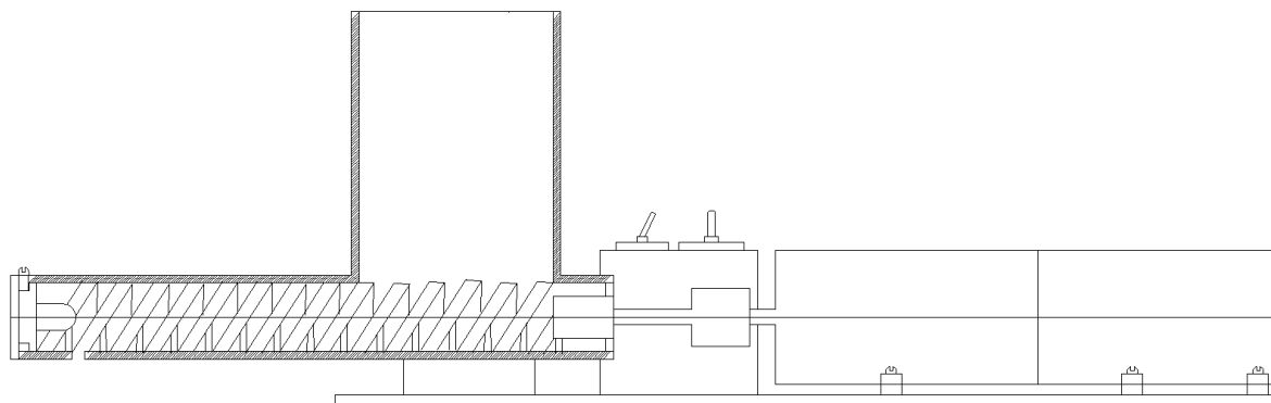
Рис. 2. Схема дозирующего устройства шнекового типа
