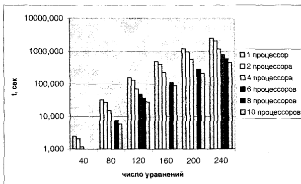
Рис. 5. Время решения систем уравнений на разных количествах процессоров
