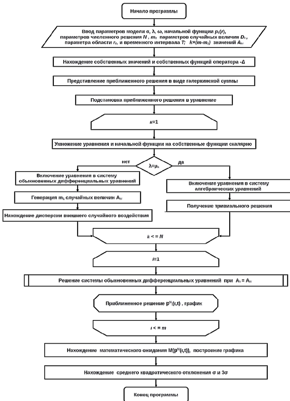
Алгоритм численного исследования стохастической модели Баренблатта–Желтова–Кочинной
