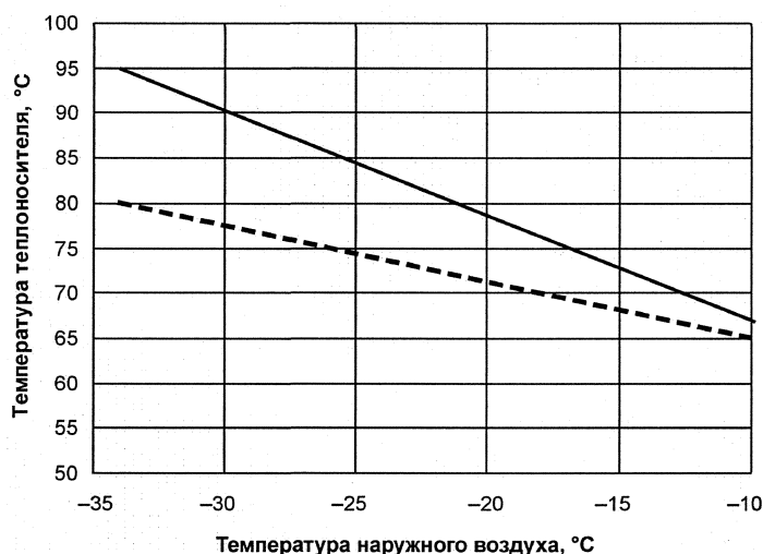
Рис. 8. Рекомендуемый ЧТС (сплошная линия) и адаптированный (штриховая линия) графики подачи
