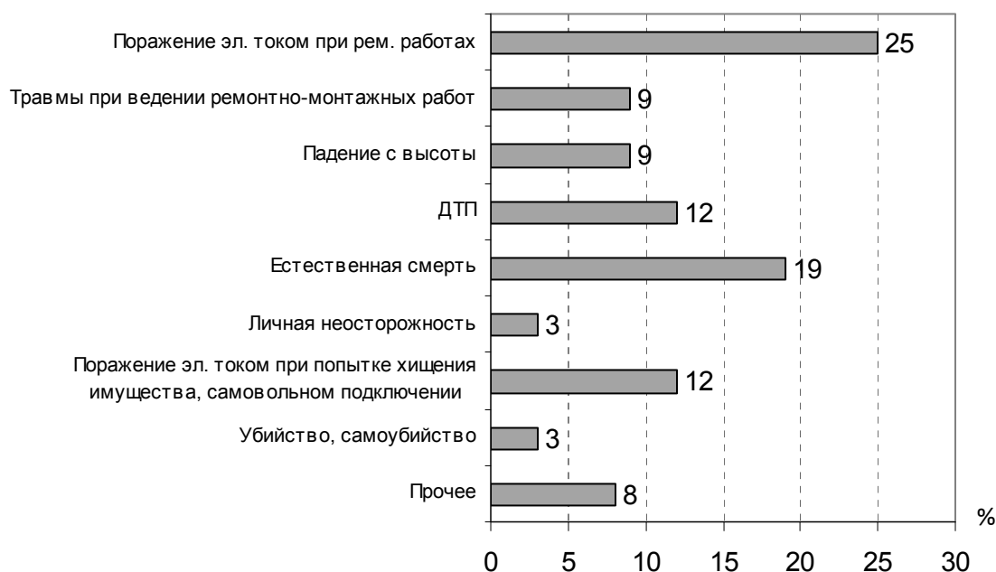
Рис. 1. Распределение причин, приводящих к смертельным несчастным случаям в электроэнергетике за 2002–2009 годы
