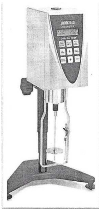
Рисунок 5. Прибор для определения вязкости.
