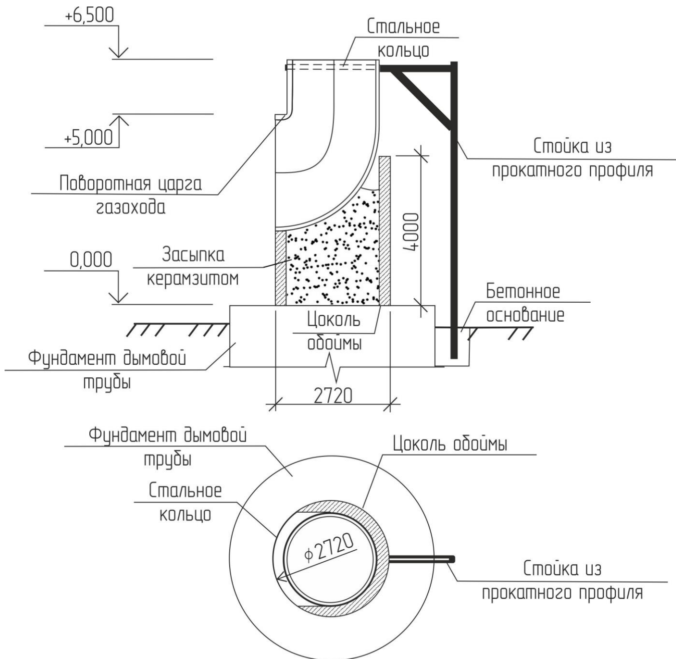
Рисунок 32. Устройство цоколя монолитной обоймы и поворотной царги газохода.
