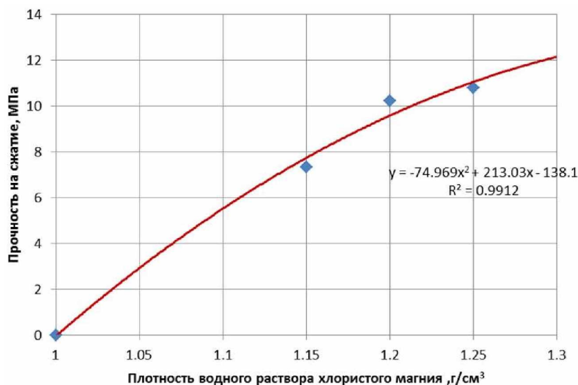
Рис. 3. Математическая зависимость прочности на сжатие магнезиального бетона от плотности затворителя при температурах выдерживания от -10 до -20 °С
