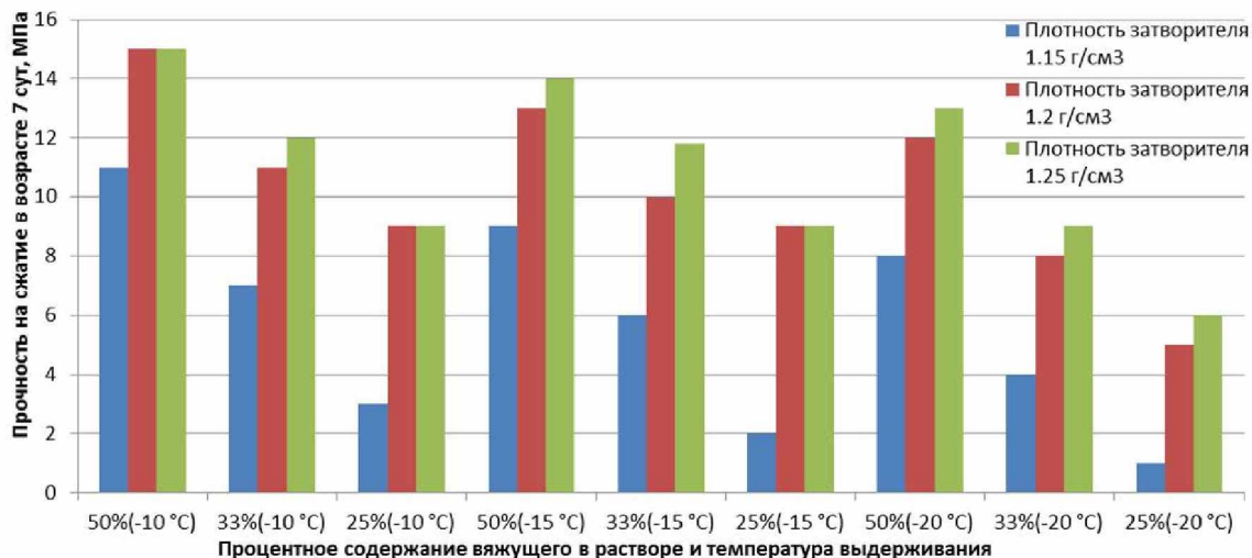
Рис. 1. Прочность на сжатие образцов магниального бетона в зависимости от процентного содержания вяжущего в материале и температуры выдерживания
