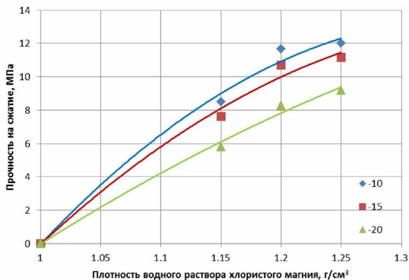
Рис. 2. Зависимость прочности на сжатие магниального бетона от плотности затворителя при различных температурах выдерживания
