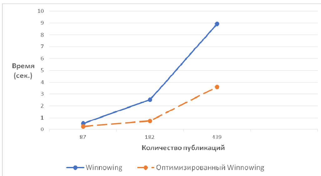
Рис. 1. Сравнительный анализ производительности алгоритмов Fig. 1. Comparative analysis of algorithms performance
