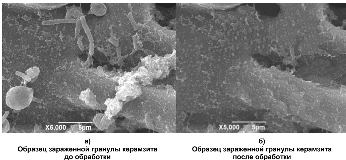
Рис. 3. Микрофотографии гранул керамзита, увеличение \times 5000
