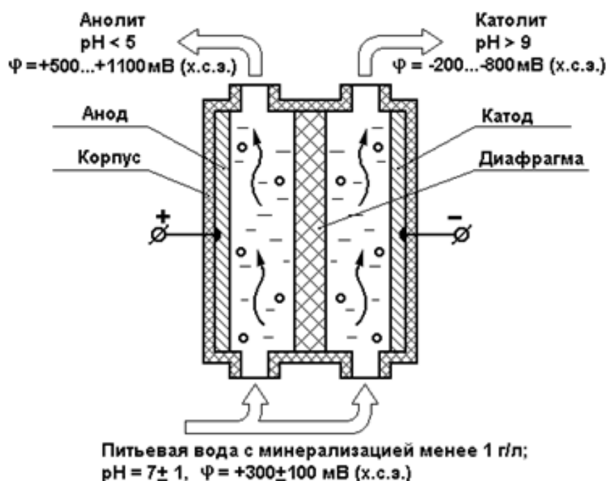
Рис. 1. Принципиальная схема устройства модуля ЭХА
