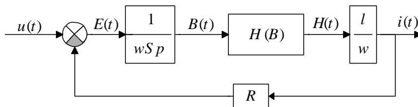
Рис. 1. Типовая структурная схема обмотки трансформатора
