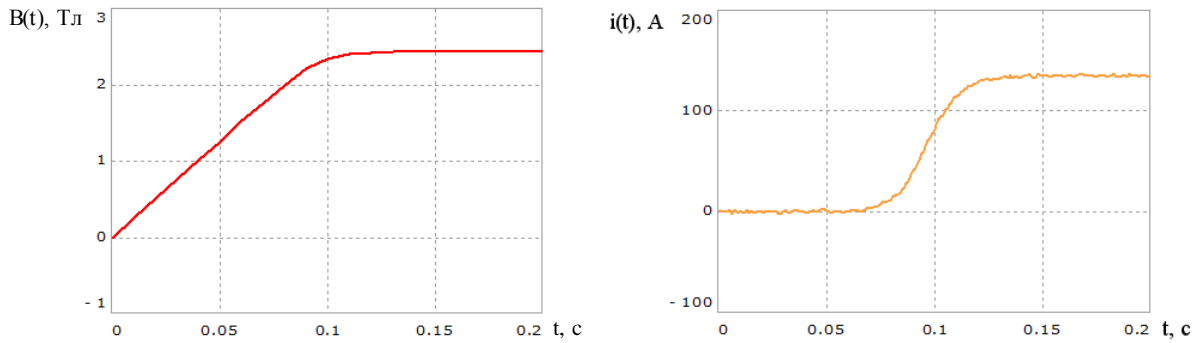
Рис. 3. Зависимость магнитной индукции и тока от времени
