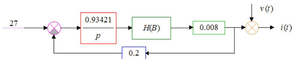
Рис. 2. Структурная схема первичной обмотки трансформатора
