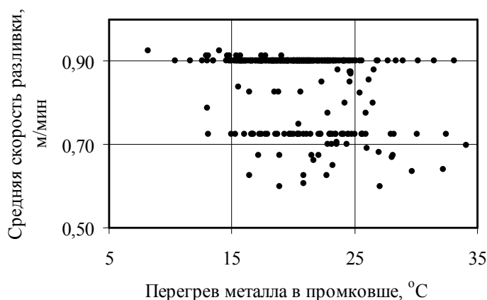
Рис. 6. Взаимосвязь скорости разливки и перегрева металла в промковше для заготовки 270 × 1200 мм из стали 09Г2С
