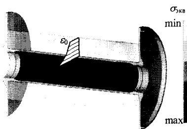
Рис. 6. МКЭ-расчет напряжений в системе «трос – барабан»
