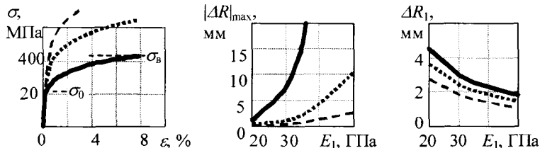
Рис. 8. Диаграммы деформирования материала барабана (а) и зависимости накопленной деформации от этих диаграмм и податливости троса (б,в)
