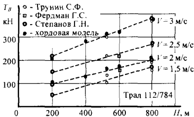
Рис. 2. Расчетные и экспериментальные зависимости усилий в ваерах от скорости и глубины буксировки трала.
