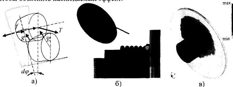
Рис. 10. Действие витка троса, завершающего слой. а) простейшая оценка, б) схема расчета МКЭ; в) распределение эквивалентных напряжений
