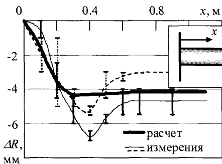
Рис. 9. Зависимость уменьшения радиуса барабана от расстояния до реборды (расчет, эксперимент).
