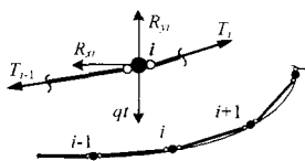
Рис. 1. Хордовая модель ваера
